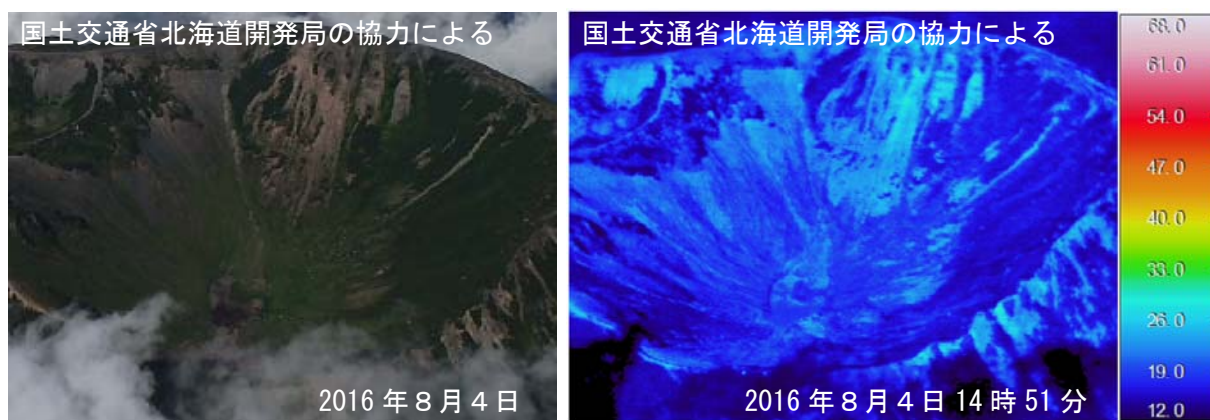
図 3 羊蹄山 赤外熱映像装置による山頂火口の地表面温度分布 図 1 中の②から撮影
