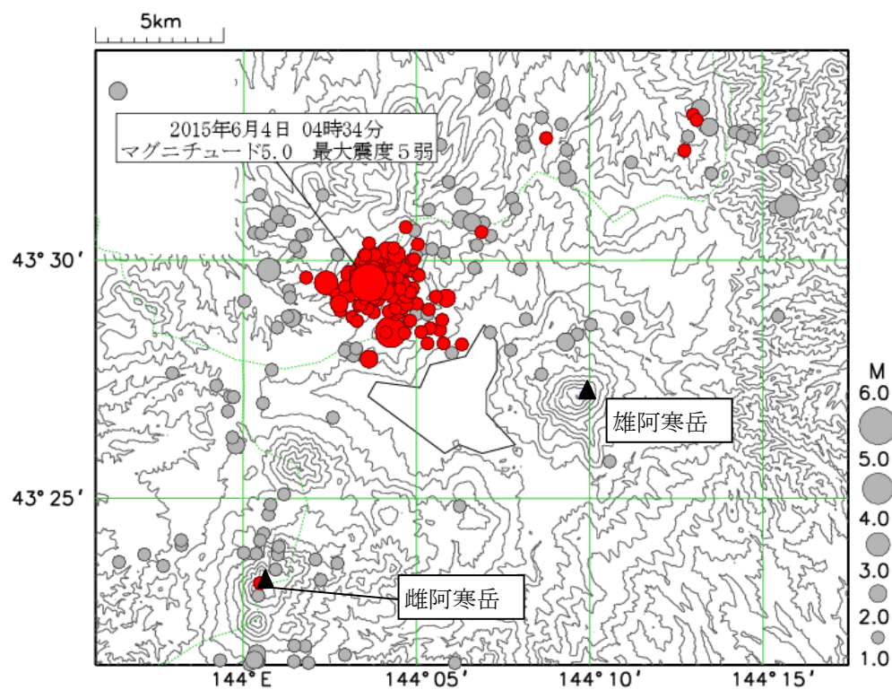
図 4 雄阿寒岳 広域地震観測網による山体周辺の地震活動 (1997 年10月 1 日～2015 年12月31日、 M \geq 1.0 、深さ30km以浅) ・ 2015 年に発生した地震を赤いシンボルで表示しています
