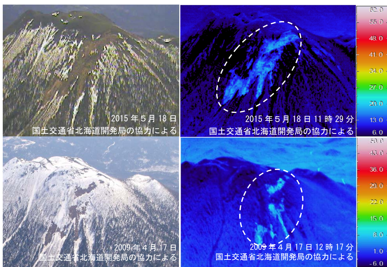
図 3 雄阿寒岳 北西側斜面の地表面温度分布 上：図 1-②の方向から撮影、下：図 1-③の方向から撮影 楕円内は北側斜面の地熱域
