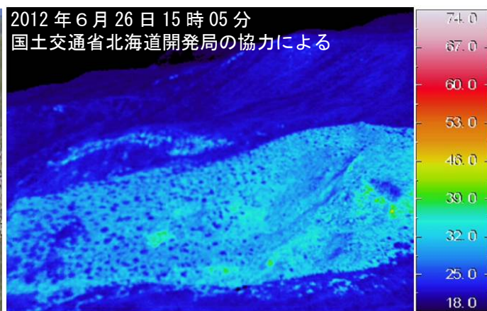
図 4 知床硫黄山 北西側中腹の爆裂火口の地表面温度分布 上：図 1-③から撮影 下：図 1-④から撮影
