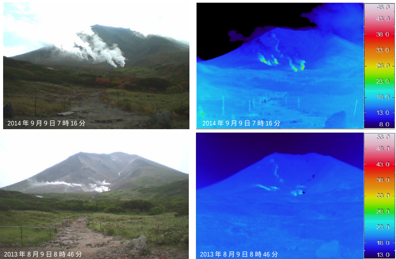
図 5 大雪山 赤外熱映像装置による旭岳地獄谷爆裂火口の地表面温度分布 東側（図 2 - ）から撮影
