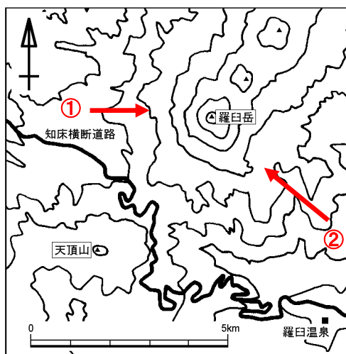
図 1 羅臼岳 周辺図
