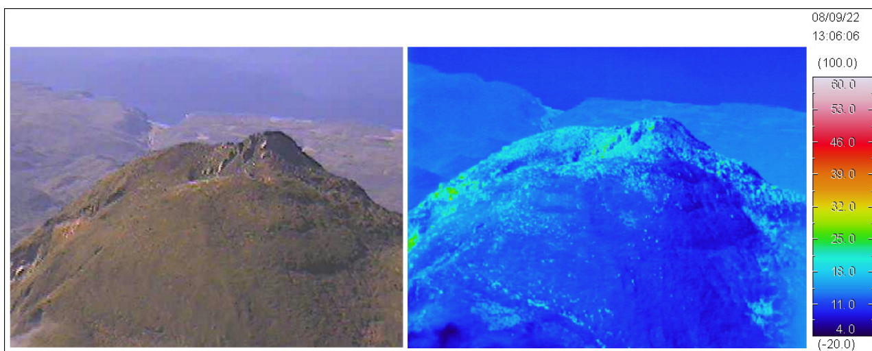
図 3 羅臼岳 赤外熱映像装置 1) による羅臼岳山頂部の地表面温度分布 (2008 年 9 月 22 日 図 1 の②方向上空より撮影)
