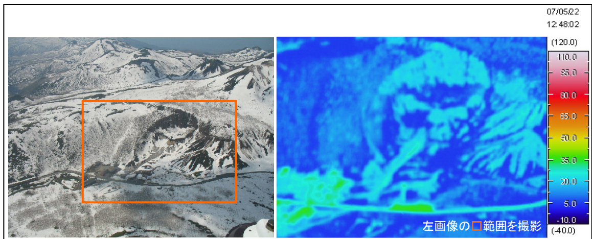
図 3 ニセコ 赤外熱映像装置 1) による五色温泉付近の地表面温度分布 (2007 年 5 月 22 日 図 2 ②方向から撮影)
