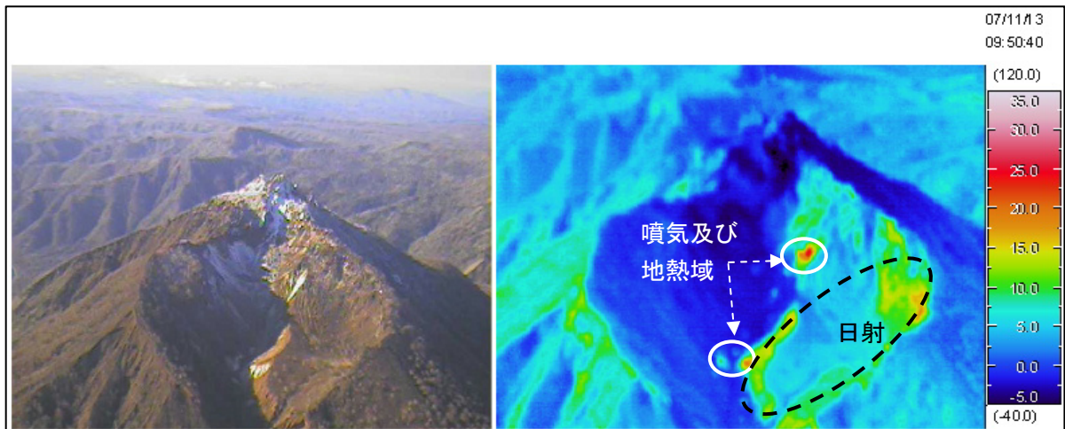
図 3 恵庭岳 赤外熱映像装置 1) による山頂爆裂火口の地表面温度分布 (2007 年 11 月 13 日 図 1 の←方向から撮影)
