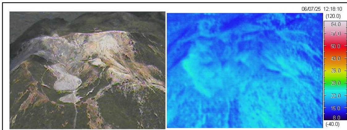
図 1 ニセコ 赤外熱映像装置*によるイワオヌプリ山頂の表面温度分布 （2006 年 7 月 25 日 南西側上空から撮影：地形図中①）
