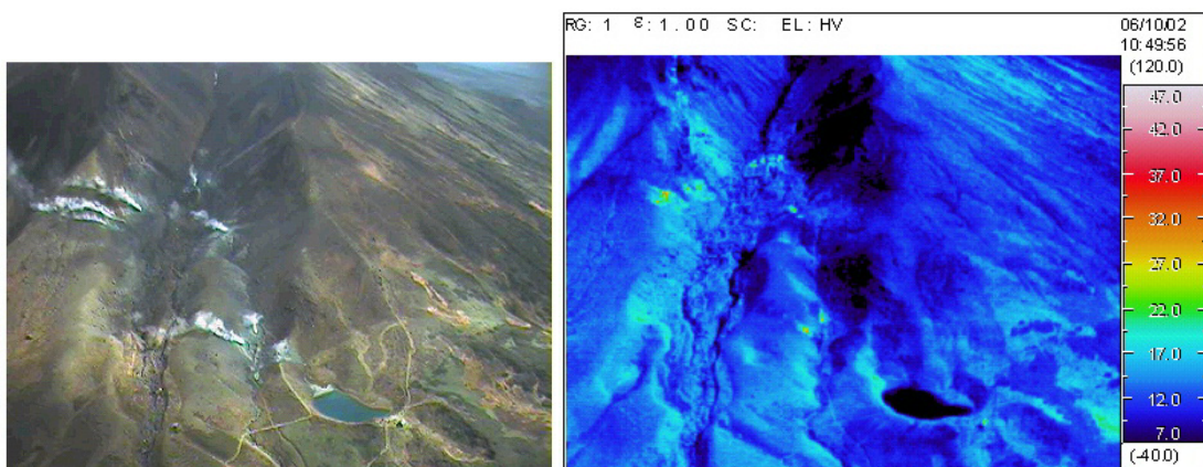
図 3 大雪山 赤外熱映像装置*による地獄谷爆裂火口の表面温度分布 （2006 年 10 月 2 日、西側上空 火口周辺図②方向から撮影）
