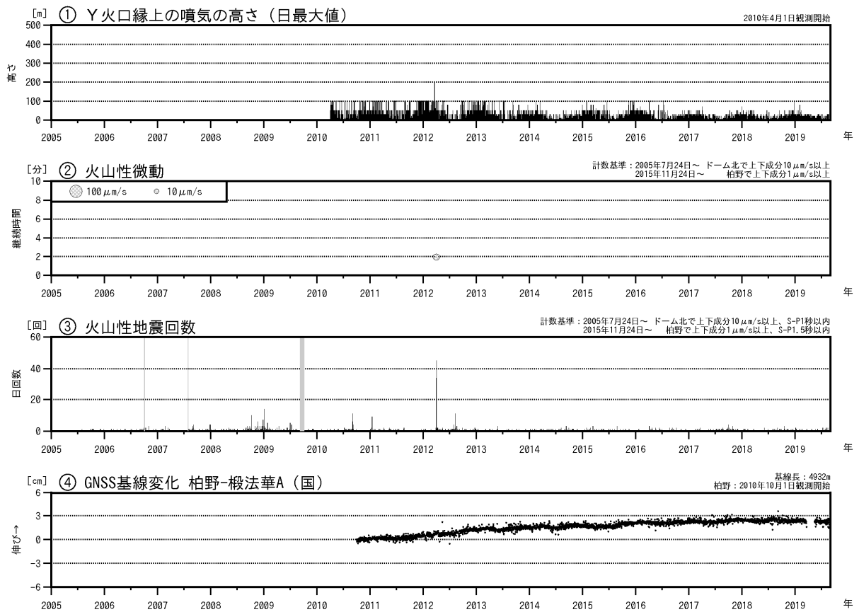
図2 恵山 火山活動経過図（2005年7月～2019年8月）
