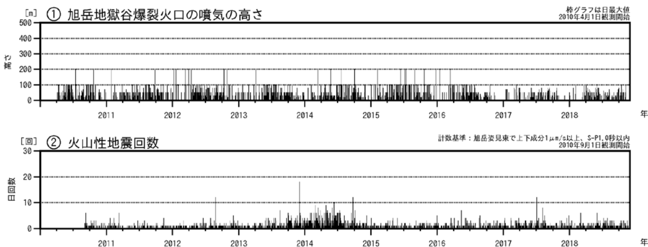
図1 大雪山 火山活動経過図（2010年4月～2018年11月）
