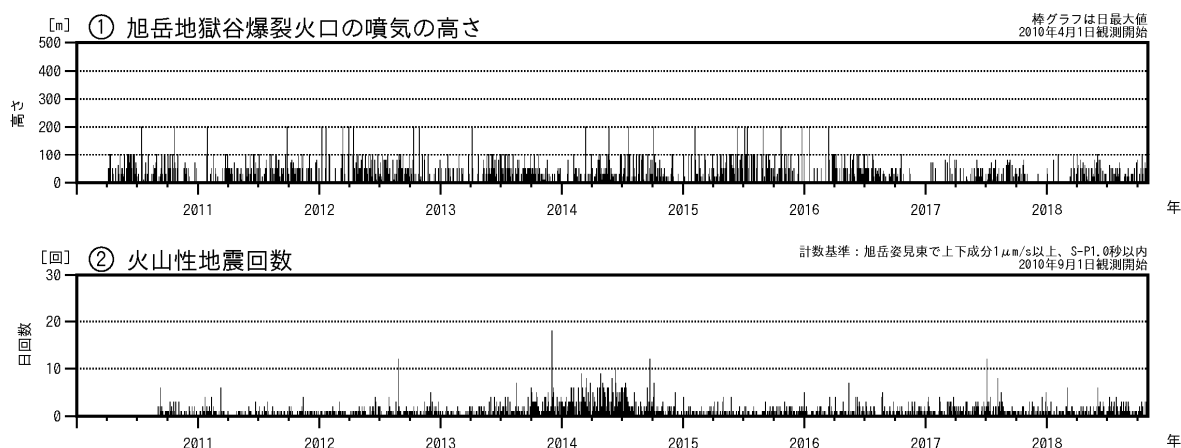
図1 大雪山 火山活動経過図（2010年4月～2018年10月）
