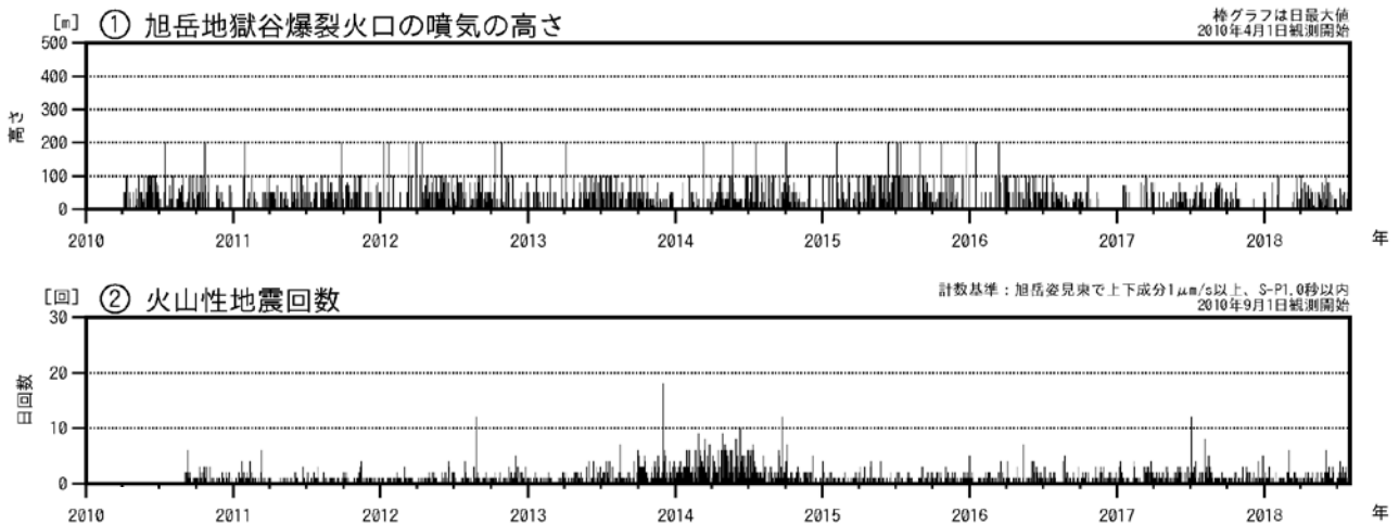
図1 大雪山 火山活動経過図（2010年4月～2018年7月）
