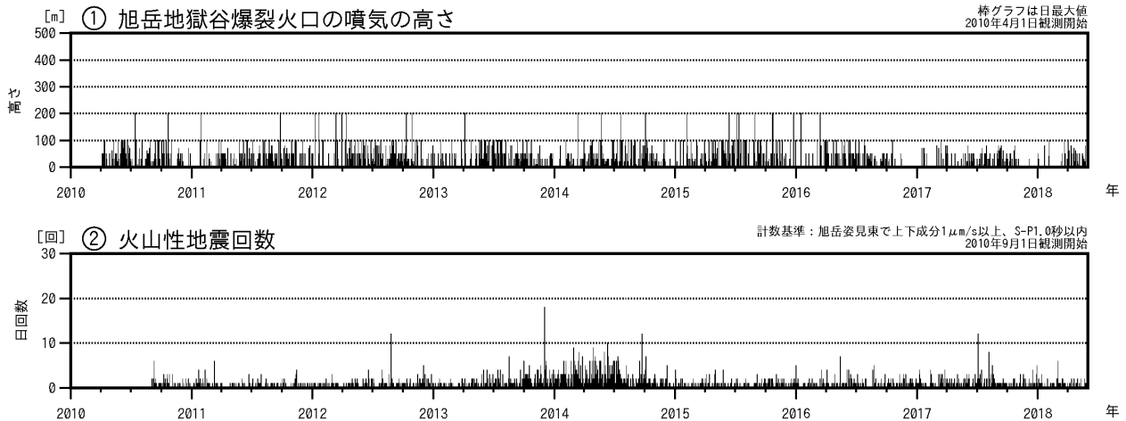
図1 大雪山 火山活動経過図（2010年4月～2018年5月）
