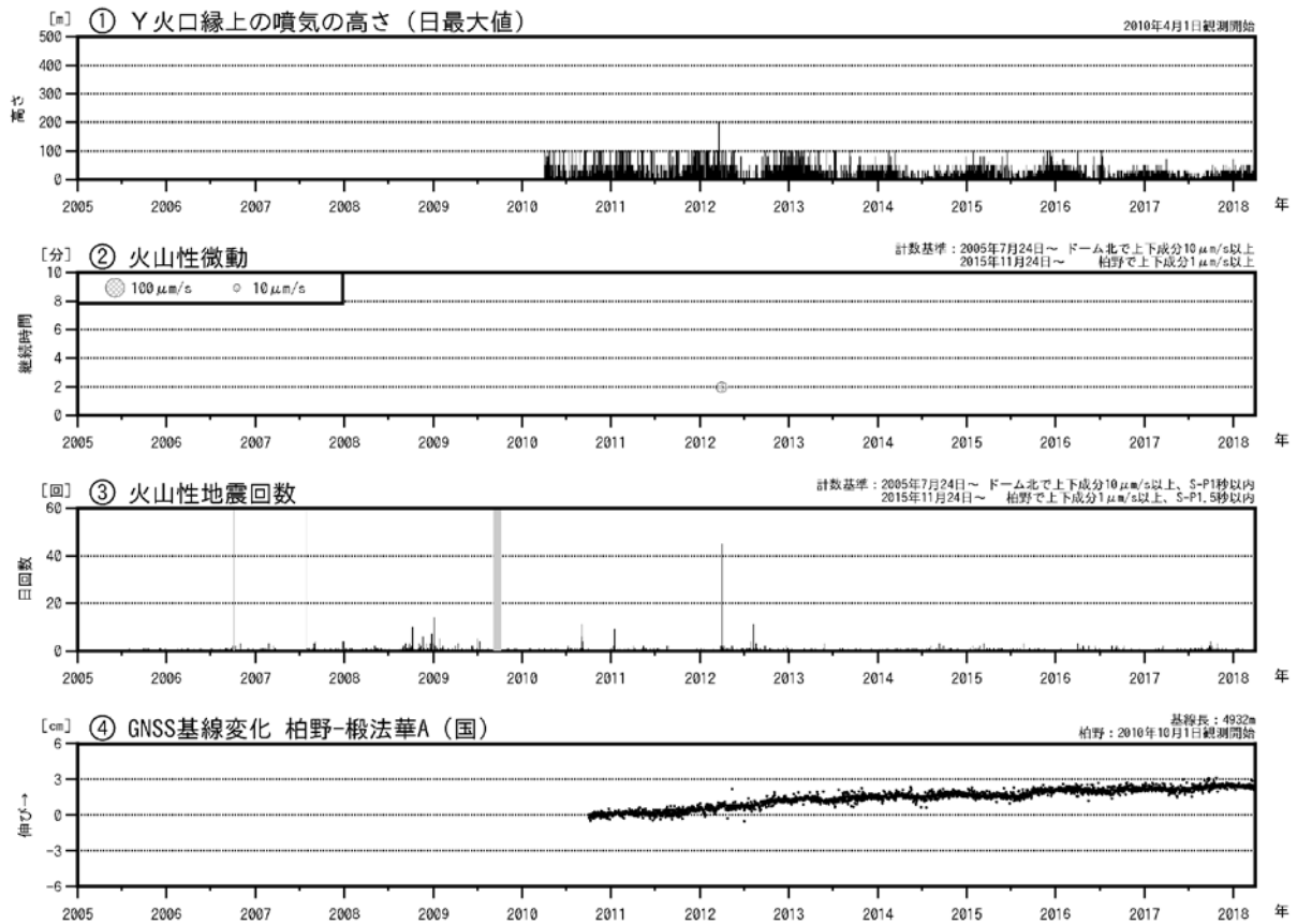
図 2 恵山 火山活動経過図（2005年 7 月～2018年 3 月）
