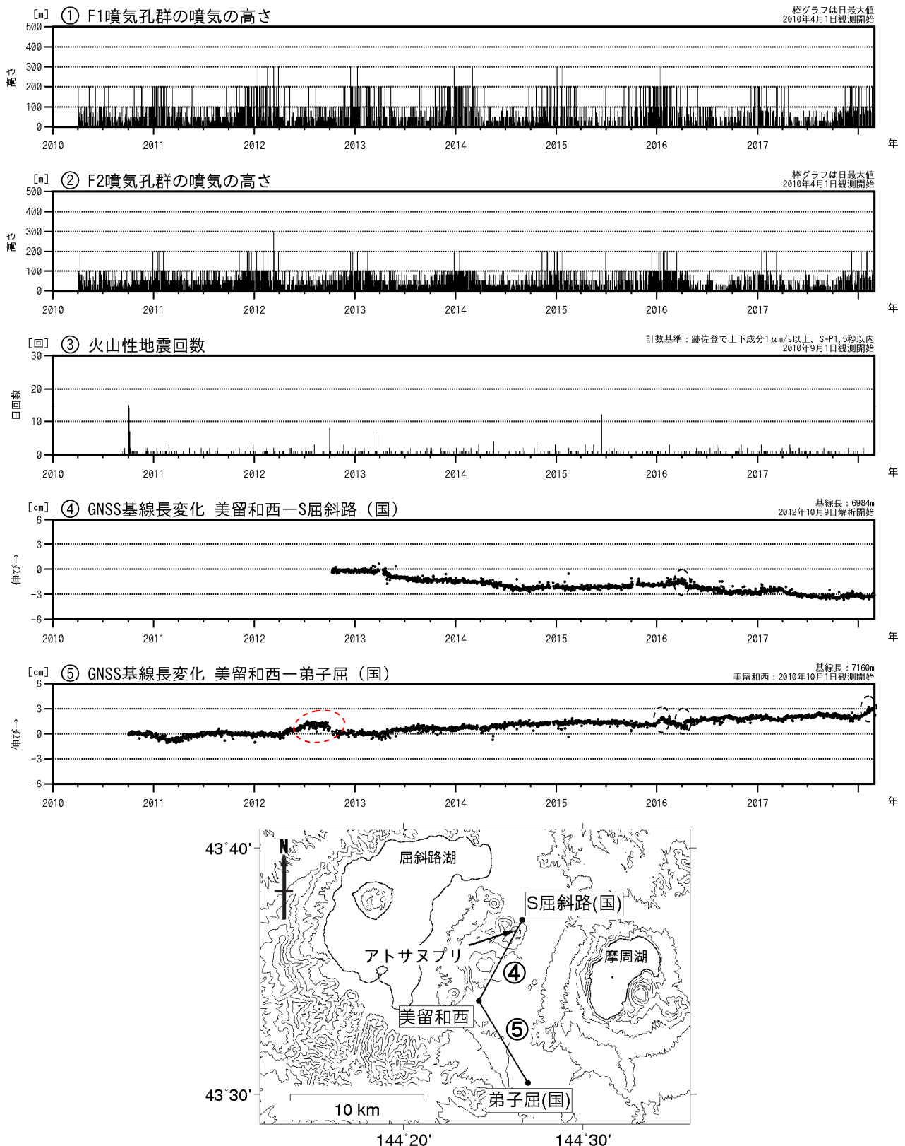
図1 アトサヌプリ 火山活動経過図（2010年4月～2018年2月）及びGNSS連続観測点配置図 ・GNSS基線の④⑤は観測点配置図の④⑤に対応しています。 ・GNSS基線の空白部分は欠測を示します。 ・④⑤の黒破線円内の変化は、美留和西観測点の局所的な動きによるもので、火山活動によるものではないと考えられます。 ・⑤の赤破線円内の変化は、弟子屈(国)付近の樹木の影響及び伐採（2012年9月下旬）によるものです。 ・(国)：国土地理院
