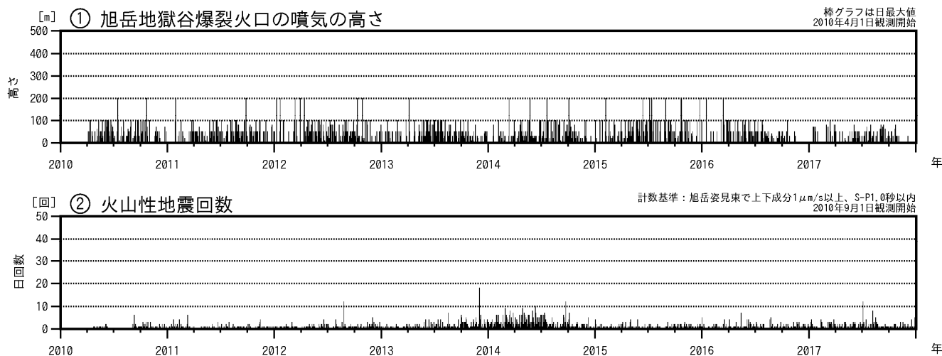
図1 大雪山 火山活動経過図（2010年4月～2017年12月）
