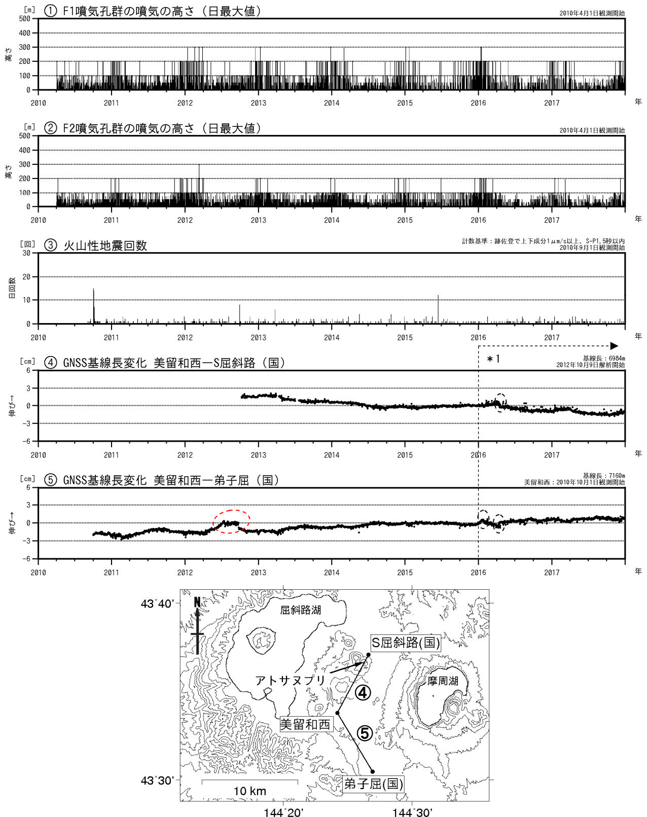
図1 アトサヌプリ 火山活動経過図 (2010年4月～2017年12月) 及びGNSS連続観測点配置図
