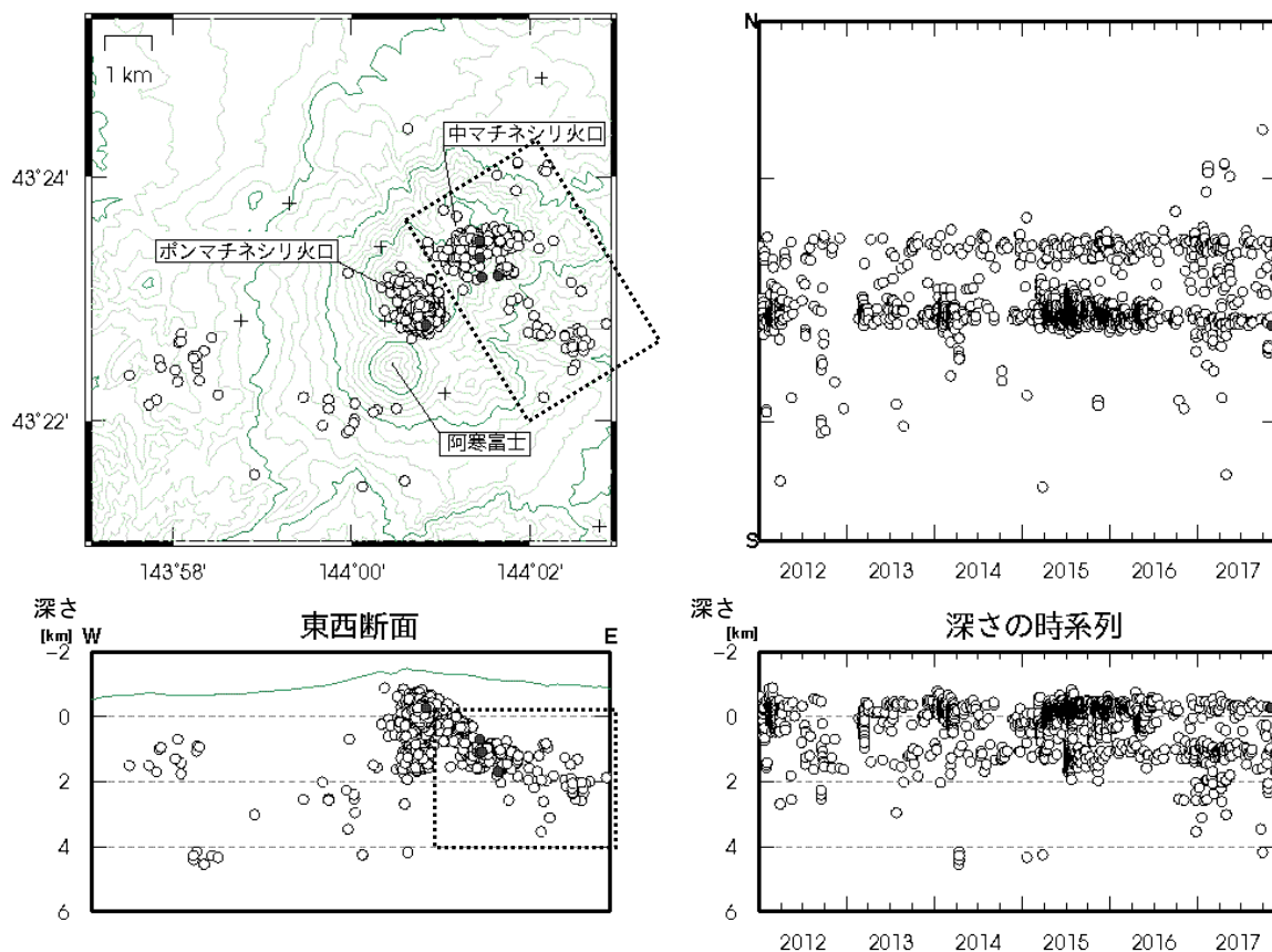
図6 雌阿寒岳 火山性地震の震源分布（2012年1月～2017年11月）
