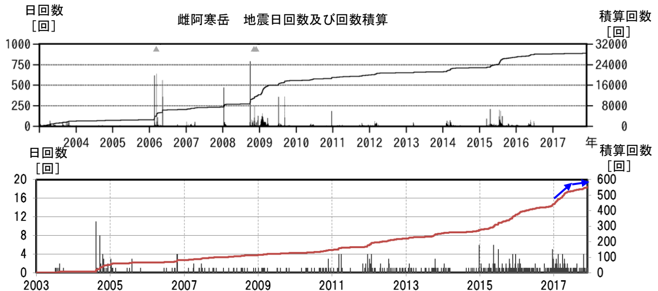
図5 雌阿寒岳 火山性地震の日回数及び積算回数推移（2003年1月～2017年11月）
