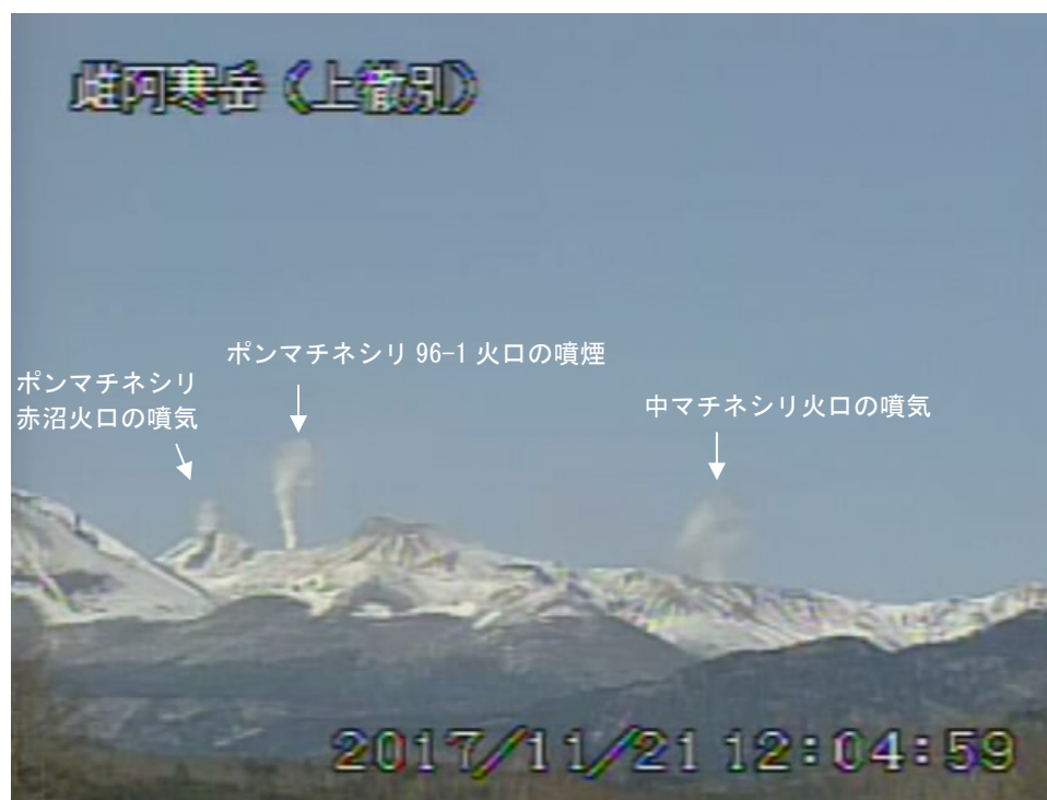
図 3 雌阿寒岳 南東側から見た山体の状況 (11月21日、上徹別監視カメラによる)
