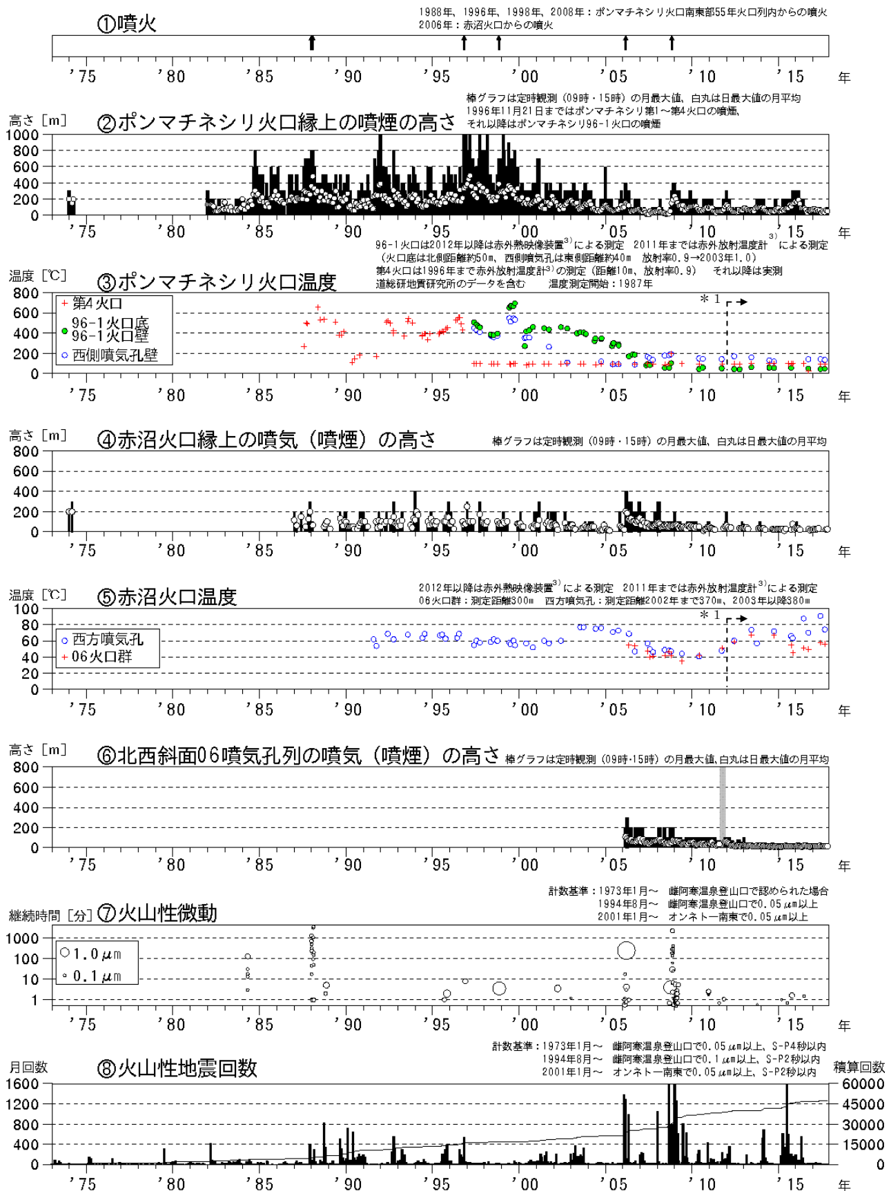
図1 雌阿寒岳 火山活動経過図（1973年1月～2017年11月）
