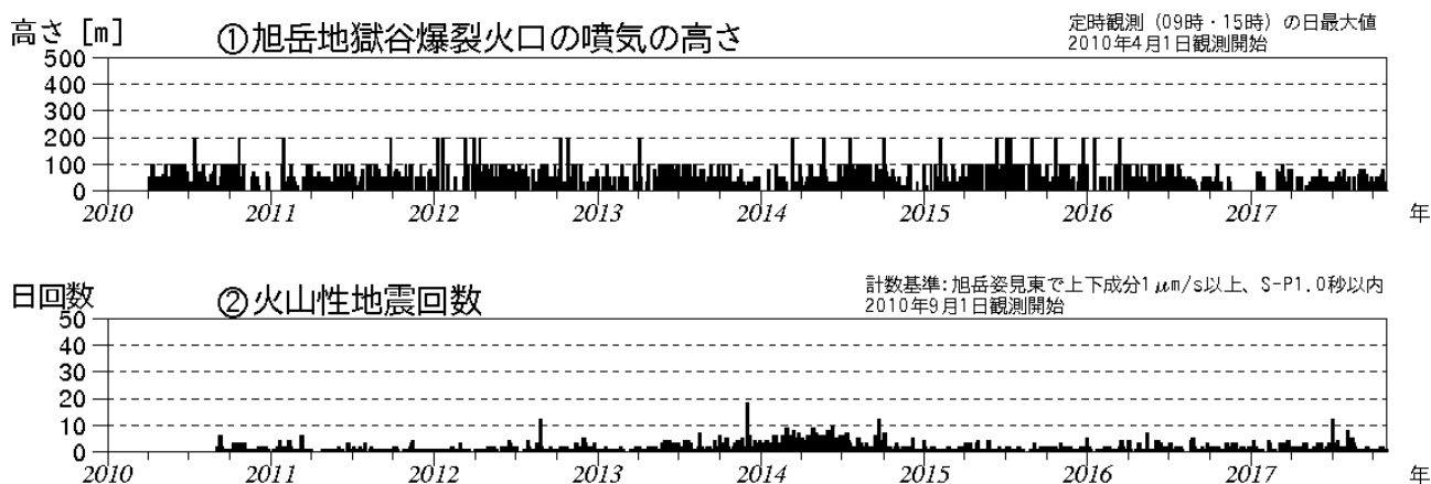
図1 大雪山 火山活動経過図（2010年4月～2017年10月）
