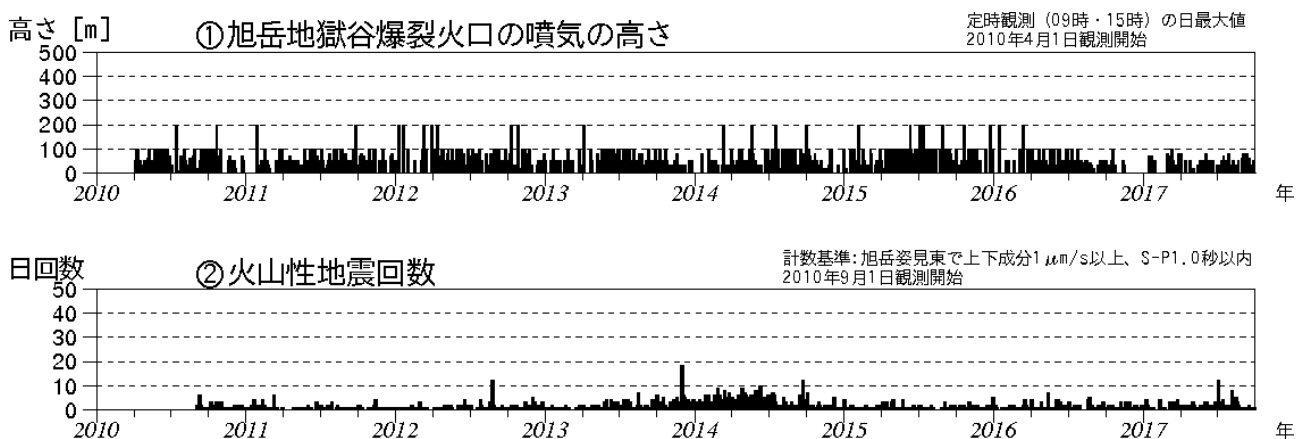
図1 大雪山 火山活動経過図（2010年4月～2017年9月）
