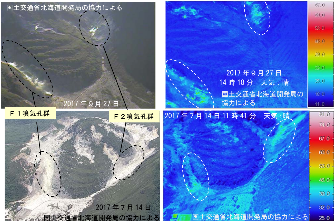
図5 アトサヌプリ F1噴気孔群及びF2噴気孔群の地表面温度分布 (上：北東側上空(図3の②)から撮影 下：北側上空(図3の③)から撮影) ・噴気の状態や地熱域(白黒破線内)に特段の変化はみられませんでした
