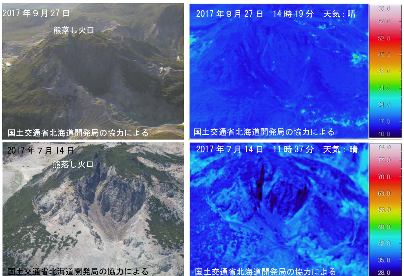
図6 アトサヌプリ 熊落し火口の地表面温度分布 北東側上空(図3の④)から撮影 ・噴気及び地熱域は確認されませんでした
