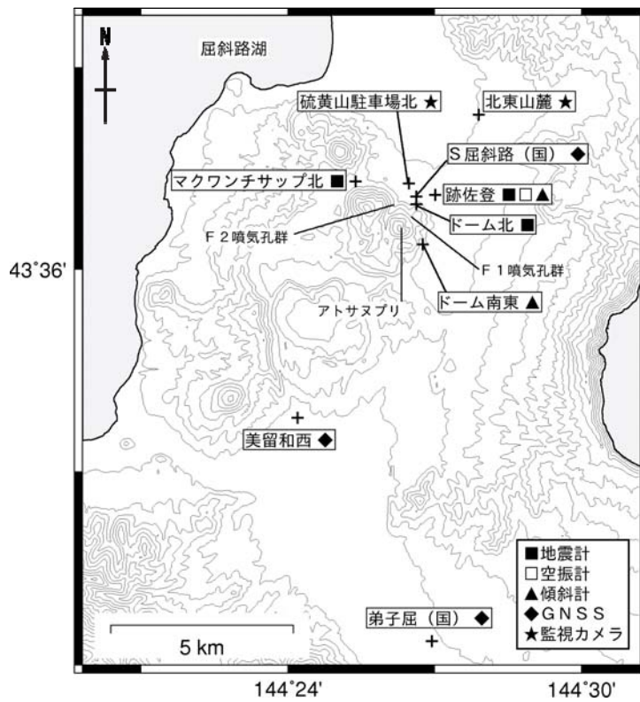
図7 アトサヌプリ 観測点配置図 +印は観測点の位置を示します 気象庁以外の機関の観測点には以下の記号を付しています (国) : 国土地理院
