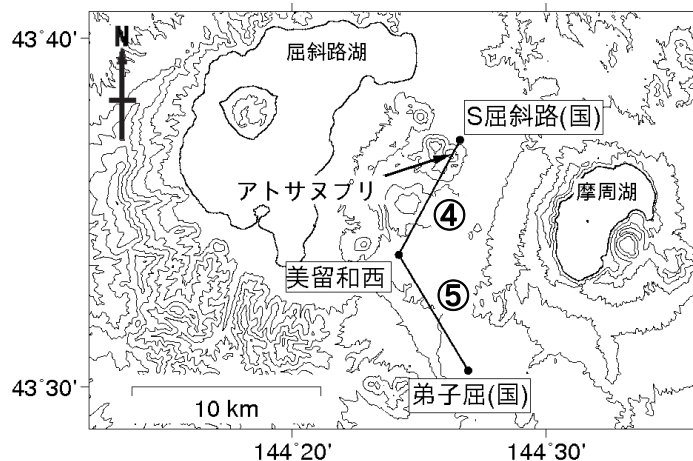
図1 アトサヌプリ 火山活動経過図（2010年4月～2017年9月）及びGNSS連続観測点配置図 ・GNSS基線の④⑤は観測点配置図の④⑤に対応しています ・GNSS基線の空白部分は欠測を示します ・④⑤の黒破線円内の変化は、美留和西観測点の局所的な動きによるもので、火山活動によるものではないと考えられます ・⑤の赤破線円内の変化は、弟子屈(国)付近の樹木の影響及び伐採（2012年9月下旬）によるものです ・(国)：国土地理院
