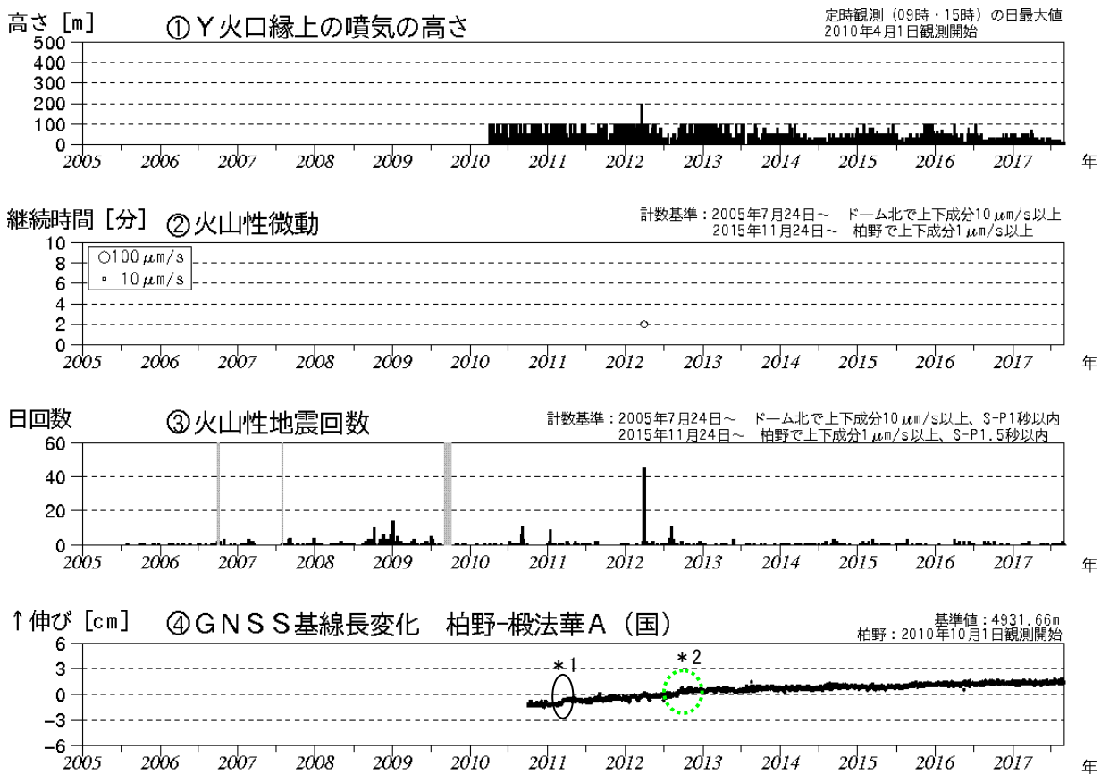
図2 恵山 火山活動経過図（2005年7月～2017年8月）
