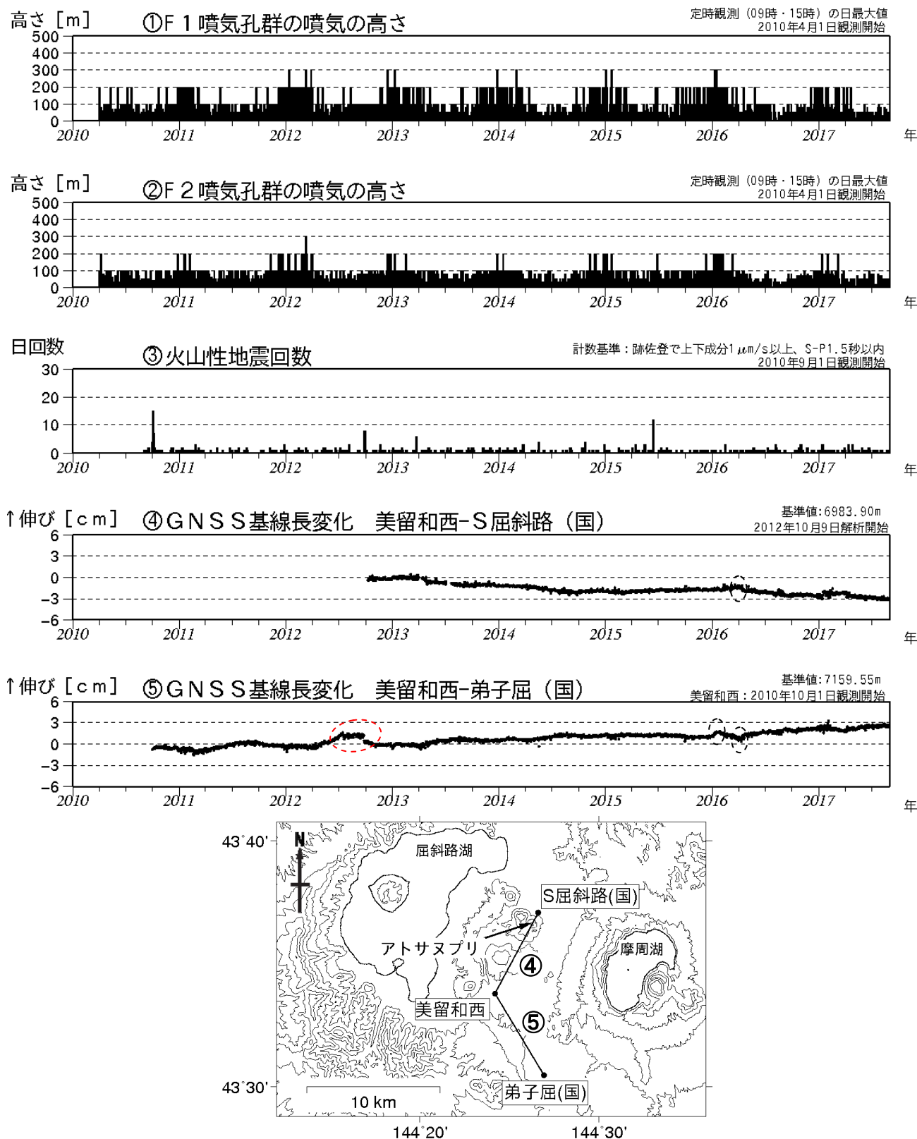
図1 アトサヌプリ 火山活動経過図（2010年4月～2017年8月）及びGNSS連続観測点配置図 ・GNSS基線の④⑤は観測点配置図の④⑤に対応しています ・GNSS基線の空白部分は欠測を示します ・④⑤の黒破線円内の変化は、美留和西観測点の局所的な動きによるもので、火山活動によるものではないと考えられます ・⑤の赤破線円内の変化は、弟子屈(国)付近の樹木の影響及び伐採（2012年9月下旬）によるものです ・(国)：国土地理院
