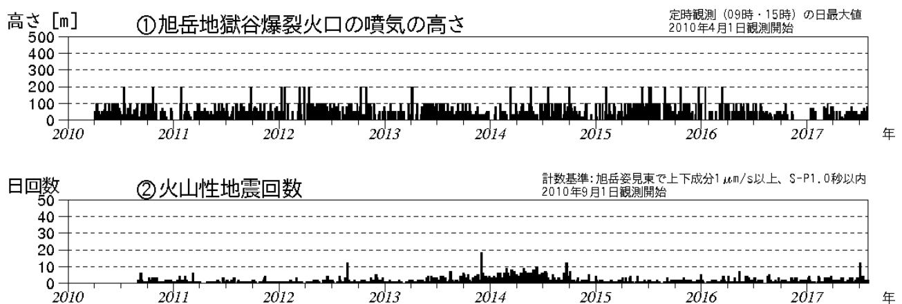
図1 大雪山 火山活動経過図（2010年4月～2017年7月）
