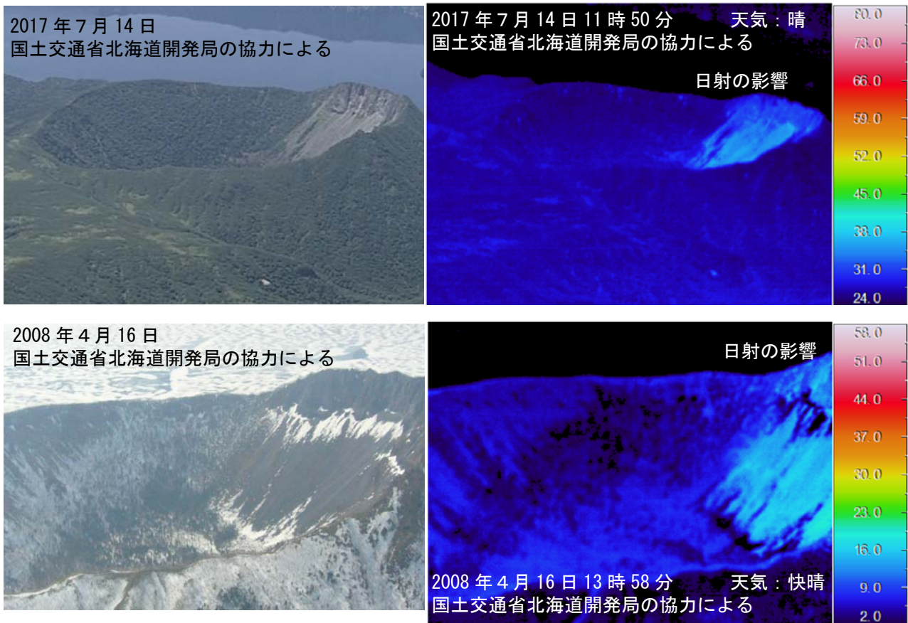
図 3 摩周 カムイヌプリの地表面温度分布 上：図 1 の②から撮影 下：図 1 の③から撮影 ・日射の影響を超える地熱域は認められませんでした
