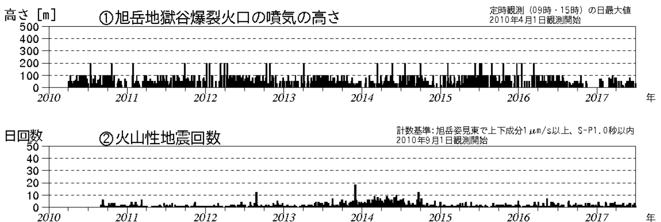
図1 大雪山 火山活動経過図（2010年4月～2017年6月）
