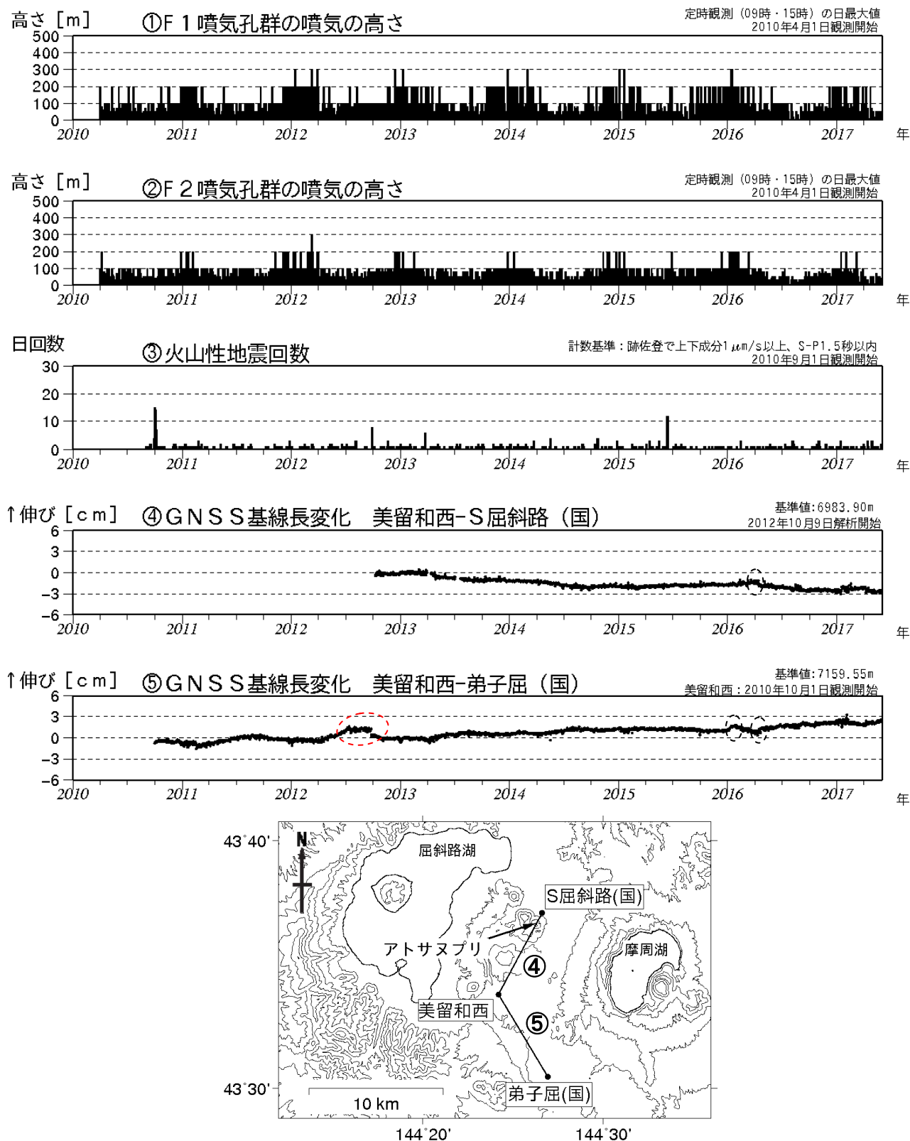
図1 アトサヌプリ 火山活動経過図（2010年4月～2017年5月）及びGNSS連続観測点配置図 ・GNSS基線の④⑤は観測点配置図の④⑤に対応しています ・GNSS基線の空白部分は欠測を示します ・④⑤の黒破線円内の変化は、美留和西観測点の局所的な動きによるもので、火山活動によるものではないと考えられます ・⑤の赤破線円内の変化は、弟子屈(国)付近の樹木の影響及び伐採（2012年9月下旬）によるものです ・(国)：国土地理院
