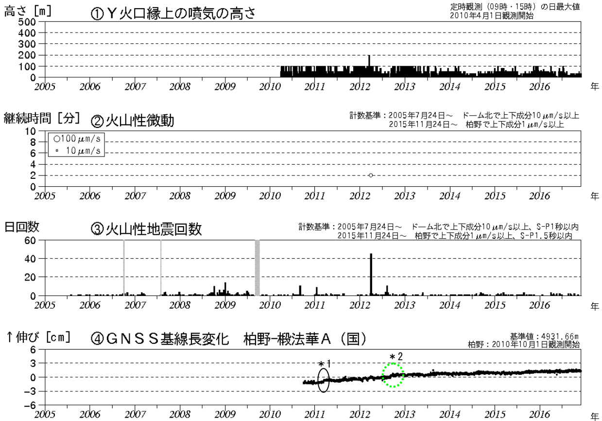
図 2 恵山 火山活動経過図（2005年 7 月～2016年11月）
