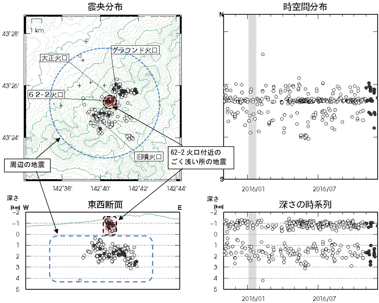
図5 十勝岳 火山性地震の震源分布 (2015年11月~2016年11月) 灰色の期間は一部観測点欠測のため震源の決定数減少や精度低下が見られます ○印: 2015年11月~2016年10月の震源 ●印: 2016年11月の震源 +印: 地震観測点
