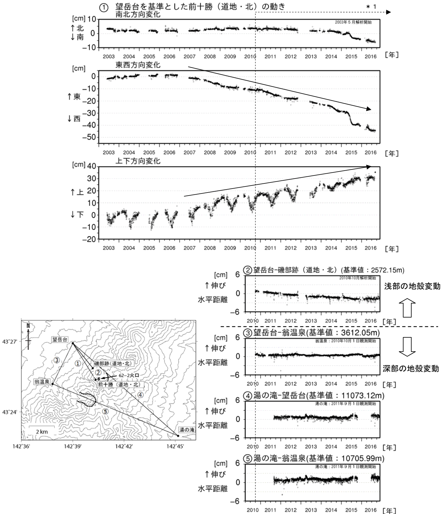
図6 十勝岳 GNSS連続観測による基線長変化（2003年5月～2016年11月）及び観測点配置図 ・GNSS基線①～⑤は観測点配置図の①～⑤に対応しています ・基線①では2006年頃から62-2火口浅部の膨張を示す前十勝観測点の動きが観測されています ・GNSS基線の空白部分は欠測を示します ・（北）：北海道大学 （道地）：地方独立行政法人北海道立総合研究機構地質研究所 * 1：2010年10月以降のデータについては、解析方法を改良して精度を向上させています
