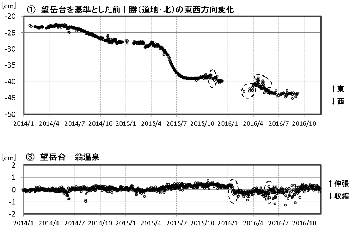
図7 十勝岳 GNSS連続観測による基線長変化拡大図 (2014年1月~2016年11月)
