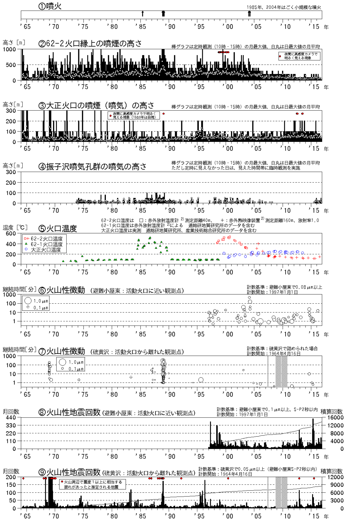
図1 十勝岳 火山活動経過図 (1964年1月~2016年11月)
