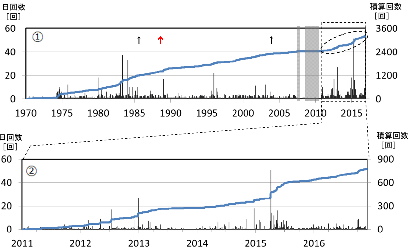
図4 十勝岳 62-2火口付近のごく浅い所の地震 (図5参照) の日回数及び積算回数推移 (上図：1970年～2016年11月 下図：2011年～2016年11月)
