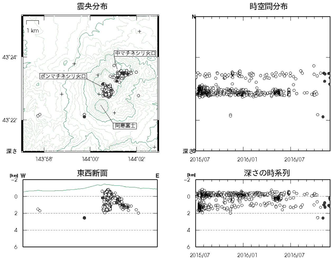
図 6 雌阿寒岳 火山性地震の震源分布（2015年7月～2016年11月）
