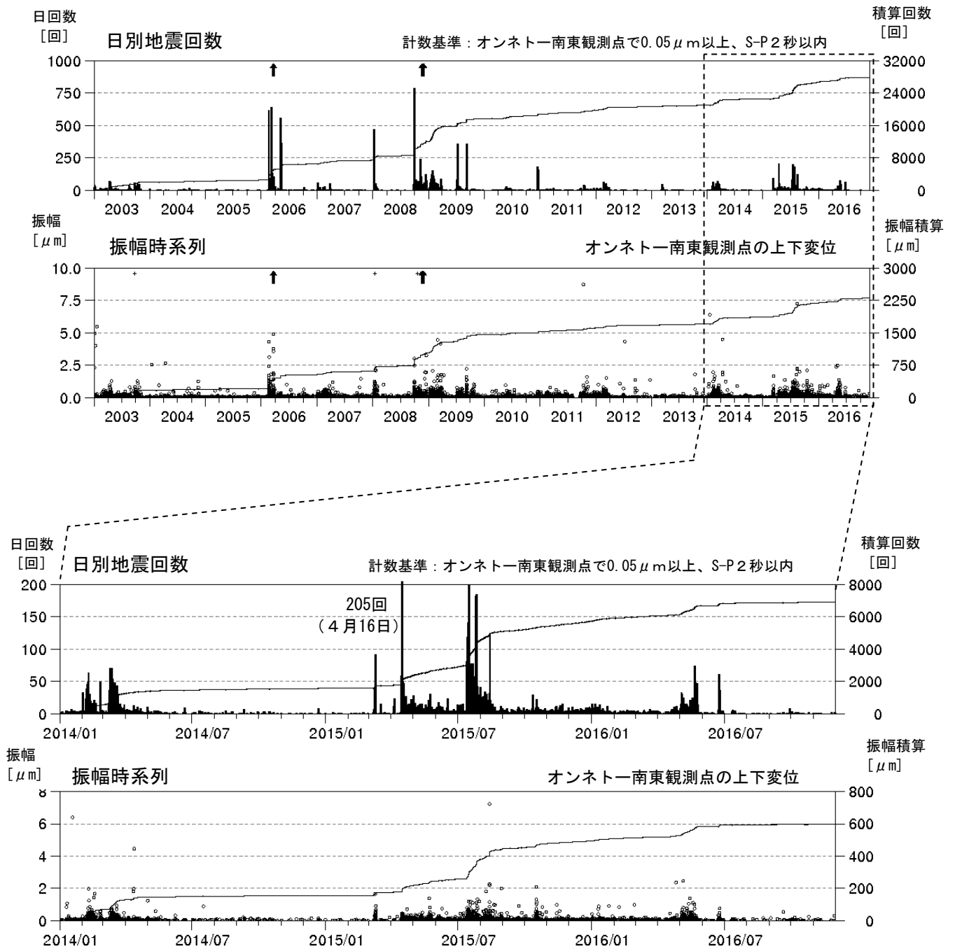
図5 雌阿寒岳 日別地震回数及び振幅時系列 上図：2003年1月1日～2016年11月30日 下図：2014年1月1日～2016年11月30日
