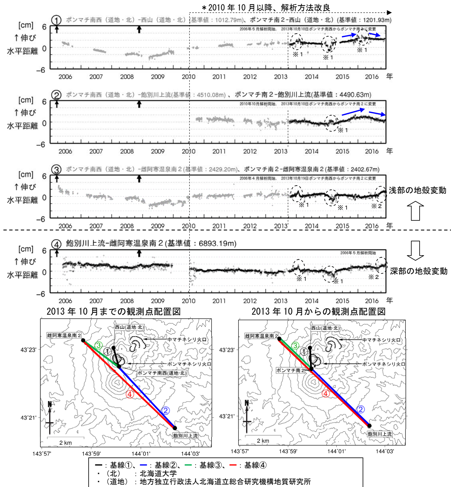
図 7 雌阿寒岳 GNSS連続観測による水平距離変化 (2006 年 4 月～2016 年 11 月) 及び観測点配置図 ・ 基線①～④は観測点配置図の①～④に対応しています ・ 基線の空白部分は欠測を示します ・ 基線図中の↑は2006年3月及び2008年11月の噴火を示します ・ 基線図中の※1 破線円内は、凍上や積雪の影響による変化を示します ・ 基線図中の※2 破線円内は、雌阿寒温泉南2の局所的な動きによるもので、火山活動によるものではないと考えられます ・ 基線①、基線②で5月頃から縮みが観測されており、ポンマチネシリ火口浅部の収縮は継続していると考えられます
