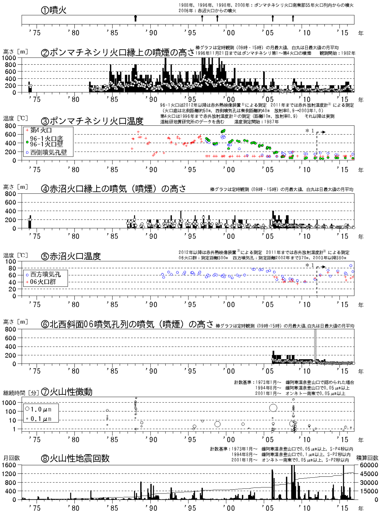
図1 雌阿寒岳 火山活動経過図（1973年1月～2016年11月）
