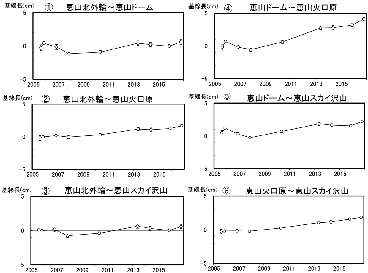
図 7 恵山 GNSS 繰り返し観測による基線長変化 (2005 年 8 月~2016 年 10 月)
