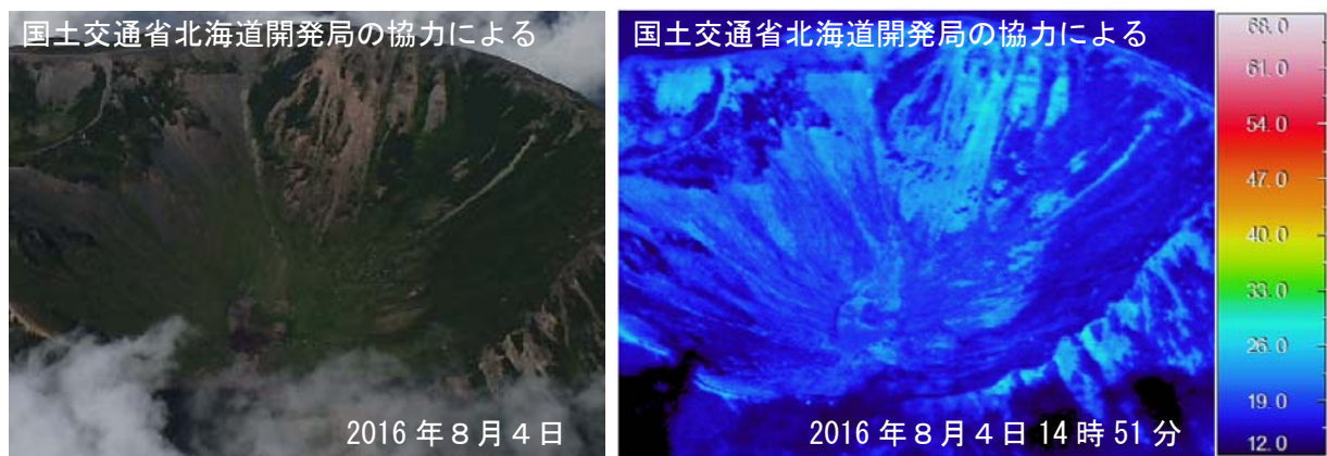
図 3 羊蹄山 赤外熱映像装置による山頂火口の地表面温度分布 図 1－②から撮影
