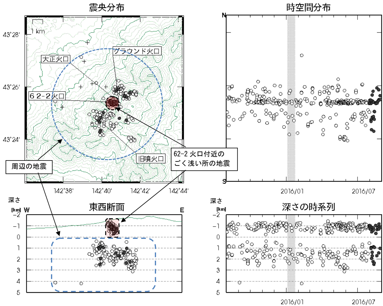
図4 十勝岳 火山性地震の震源分布（2015年8月～2016年8月） 灰色の期間は一部観測点欠測のため震源の決定数減少や精度低下が見られます ○印：2015年8月～2016年7月の震源 ●印：2016年8月の震源 +印：地震観測点
