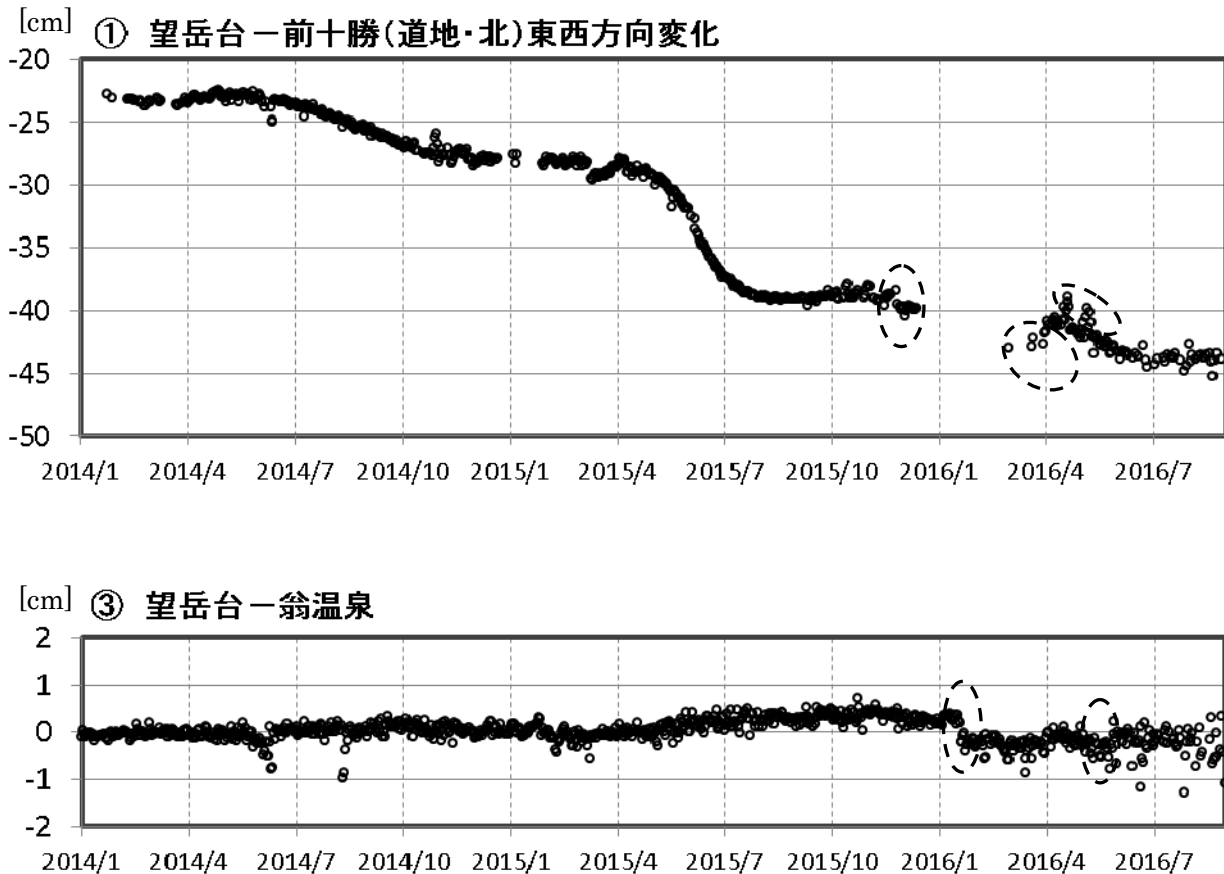
図 6 十勝岳 GNSS連続観測による基線長変化拡大図（2014年 1 月～2016年 8 月）
