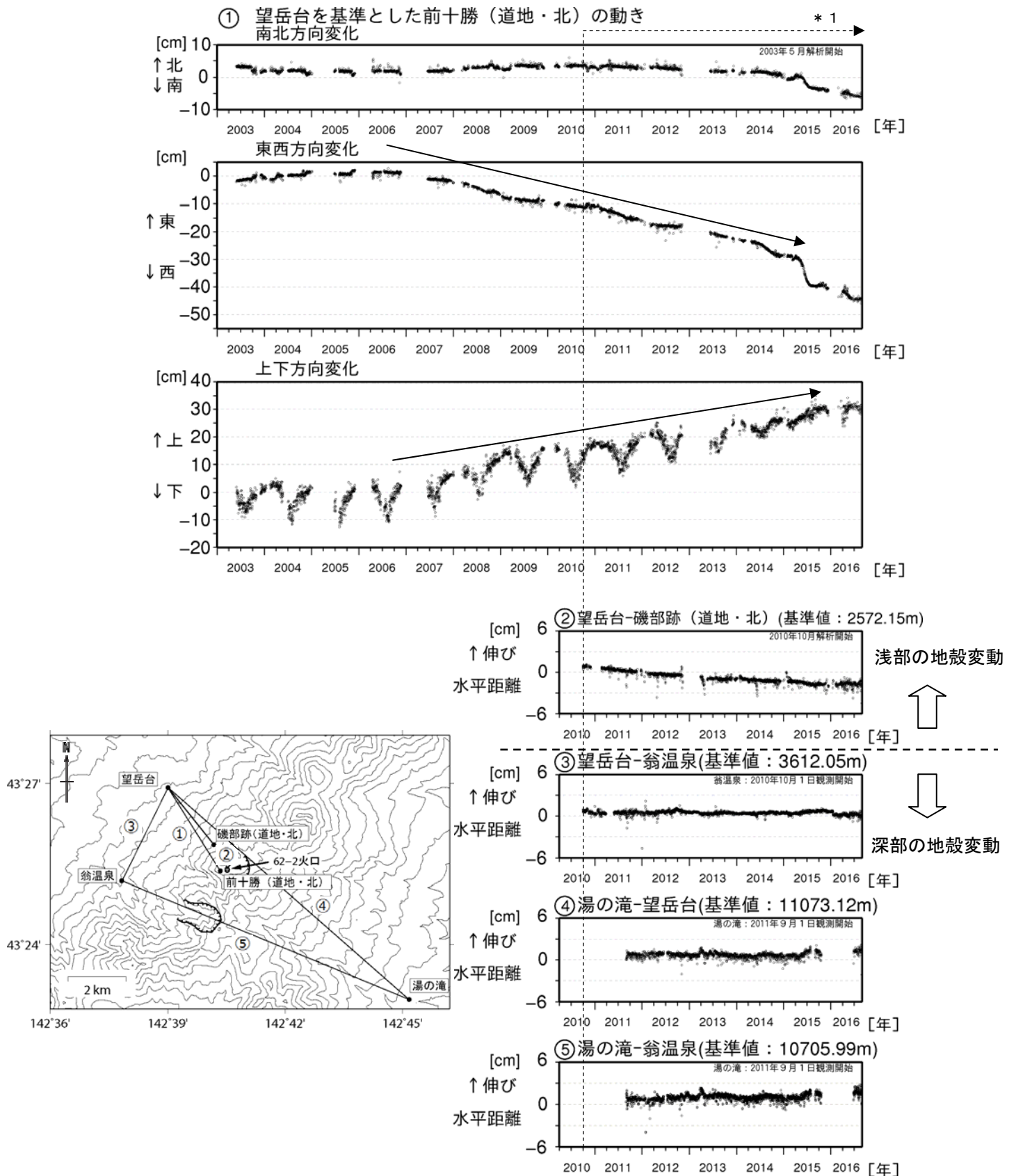
図5 十勝岳 GNSS連続観測による基線長変化（2003年5月～2016年8月）及び観測点配置図
