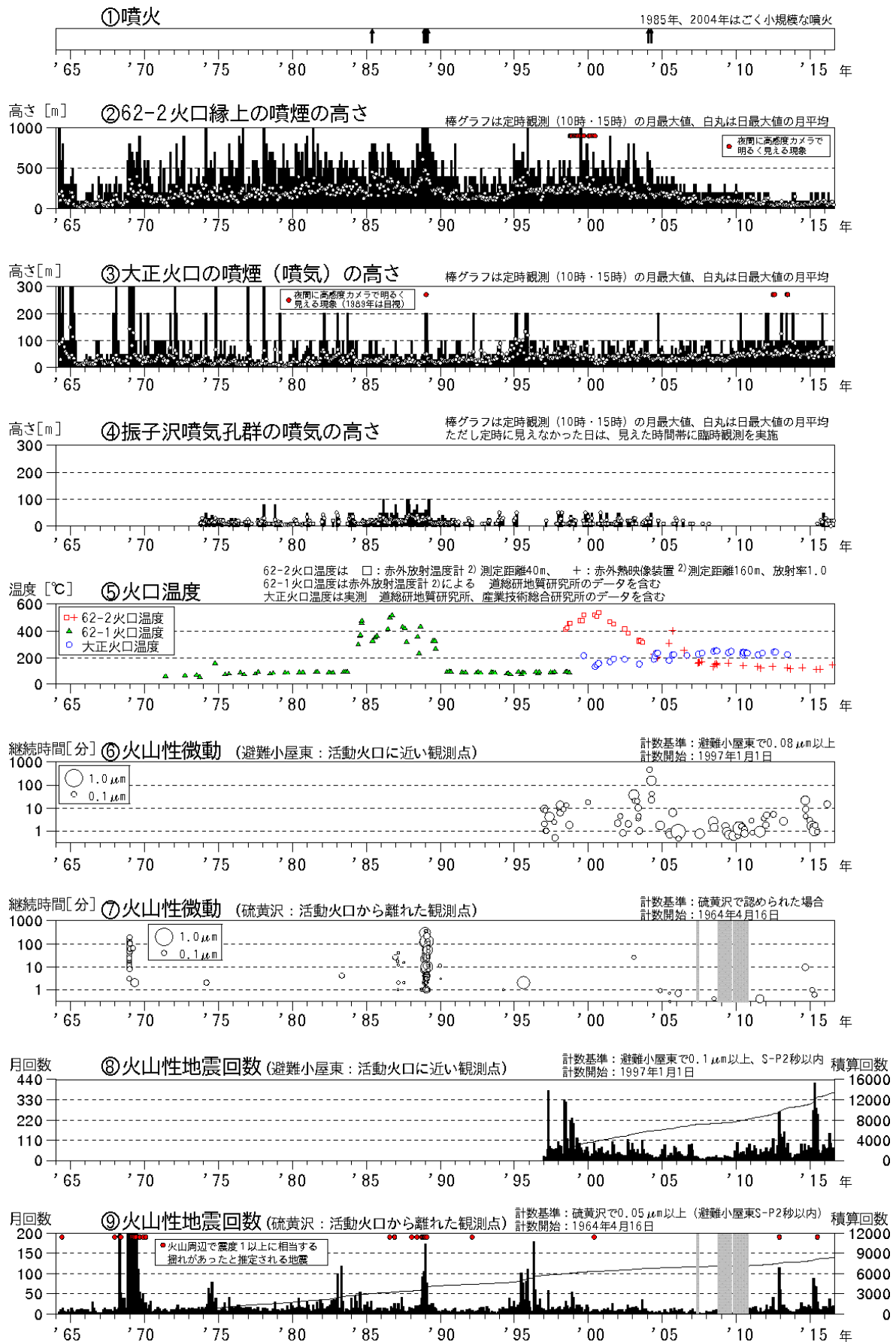
図1 十勝岳 火山活動経過図（1964年1月～2016年8月）
