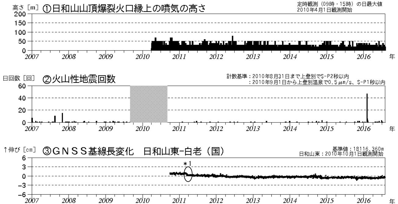
図 2 倶多楽 火山活動経過図（2007年 1 月～2016年 7 月）
