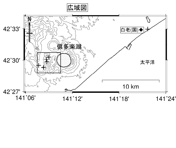
図 3 倶多楽 観測点配置図
