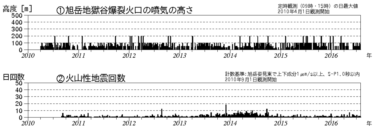
図1 大雪山 火山活動経過図（2010年4月～2016年7月）
