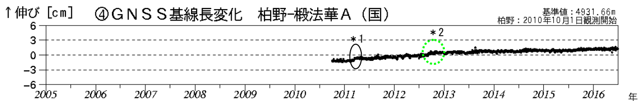
図2 恵山 火山活動経過図（2005年7月～2016年6月）
