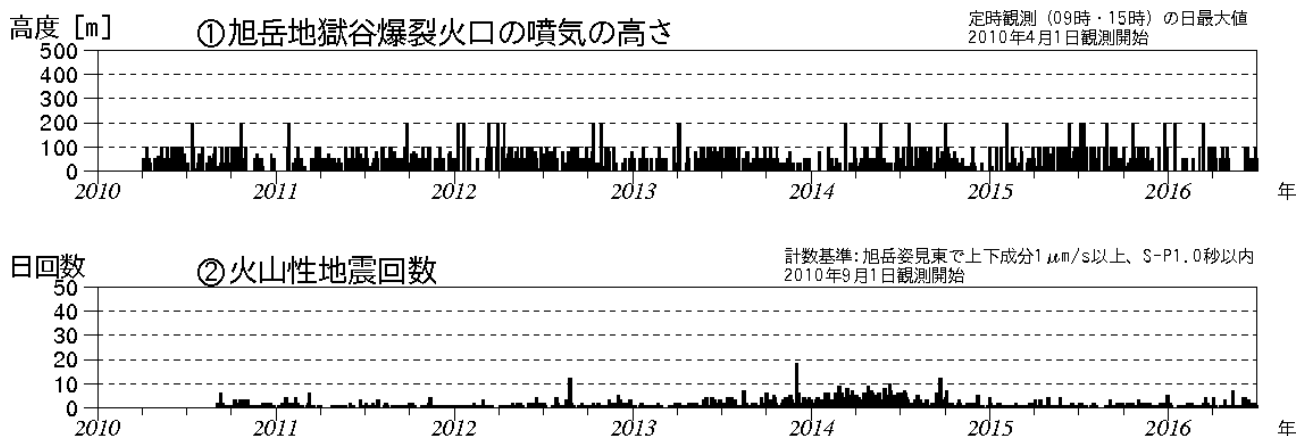
図1 大雪山 火山活動経過図（2010年4月～2016年6月）
