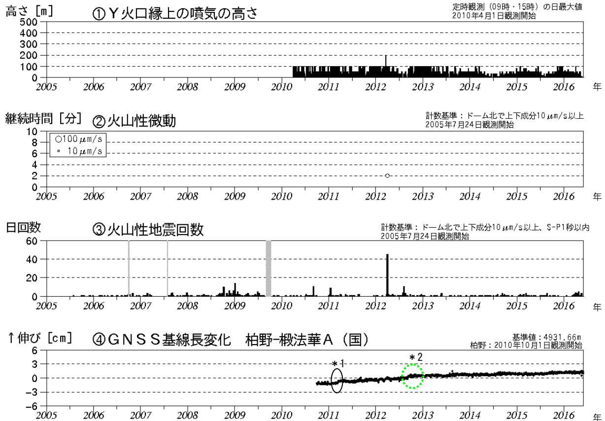
図2 恵山 火山活動経過図（2005年7月～2016年5月）
