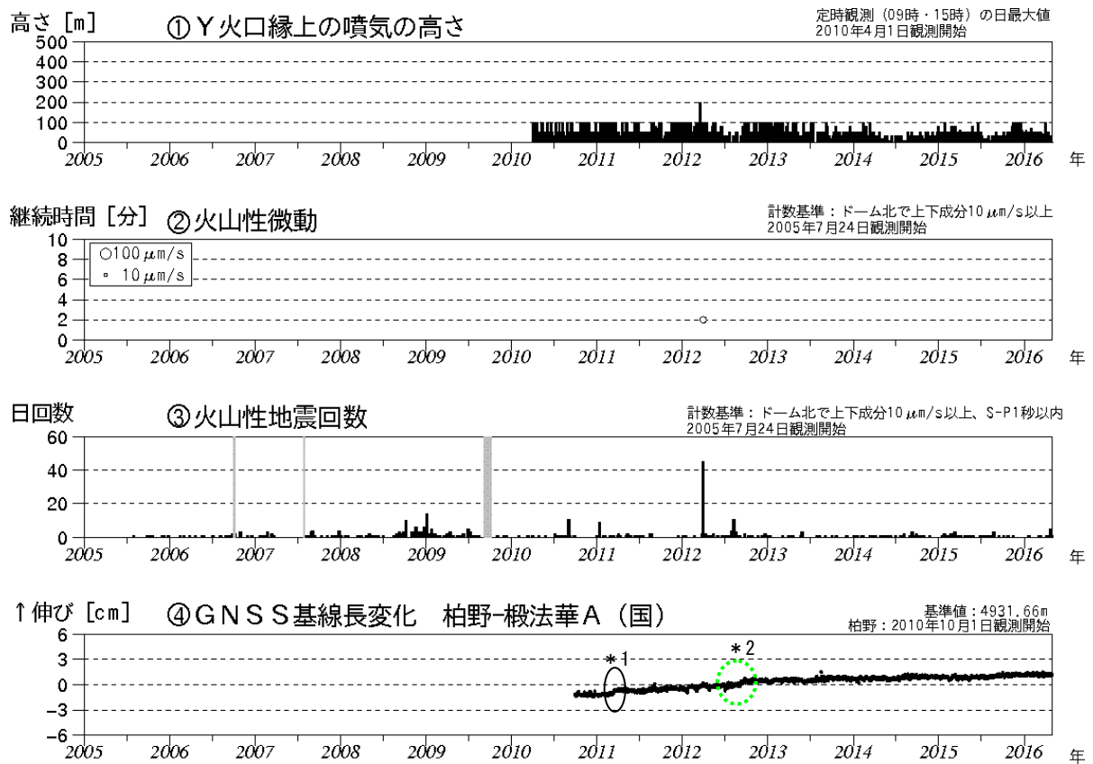
図2 恵山 火山活動経過図（2005年7月～2016年4月）
