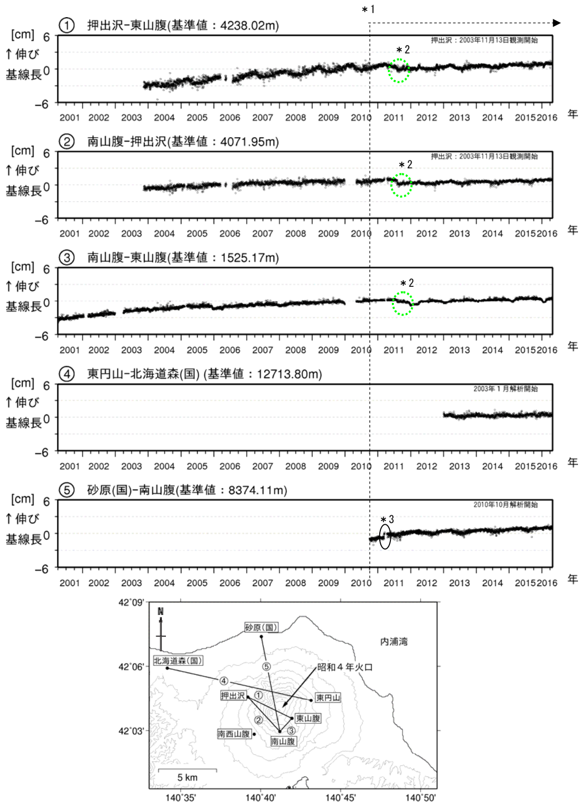
図5 北海道駒ヶ岳 GNSS連続観測による基線長変化（2001年4月～2016年4月）及び観測点配置図
