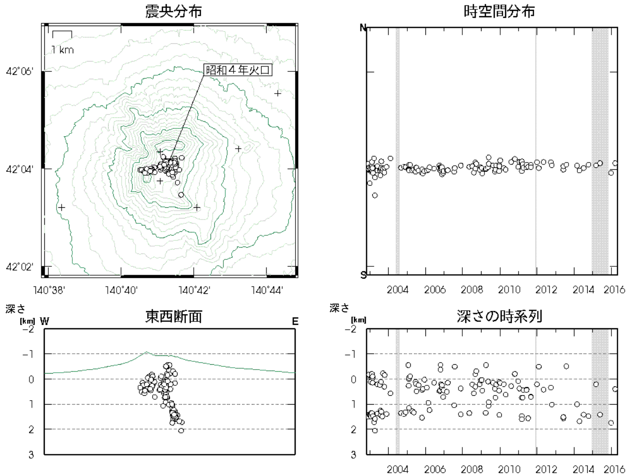
図 4 北海道駒ヶ岳 火山性地震の震源分布（2002年12月～2016年4月） 灰色の期間は一部観測点欠測のため震源の決定数減少や精度低下が見られます +印：地震観測点 ・今期間、震源が決定された地震はありませんでした
