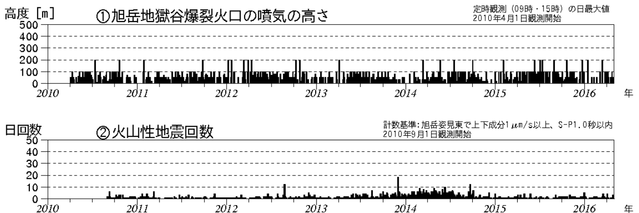
図 1 大雪山 火山活動経過図（2010年 4 月～2016年 4 月）
