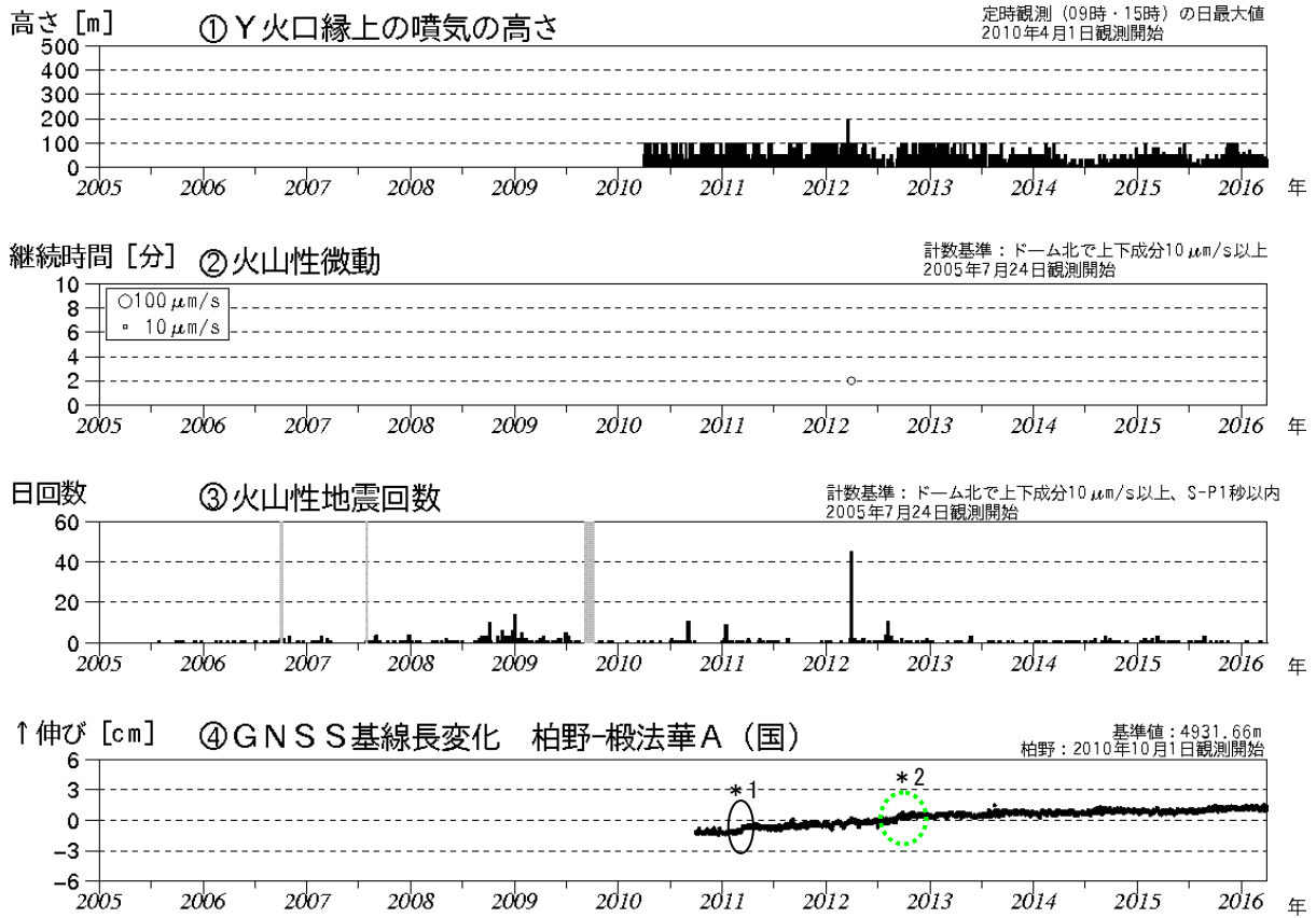
図2 恵山 火山活動経過図（2005年7月～2016年3月）
