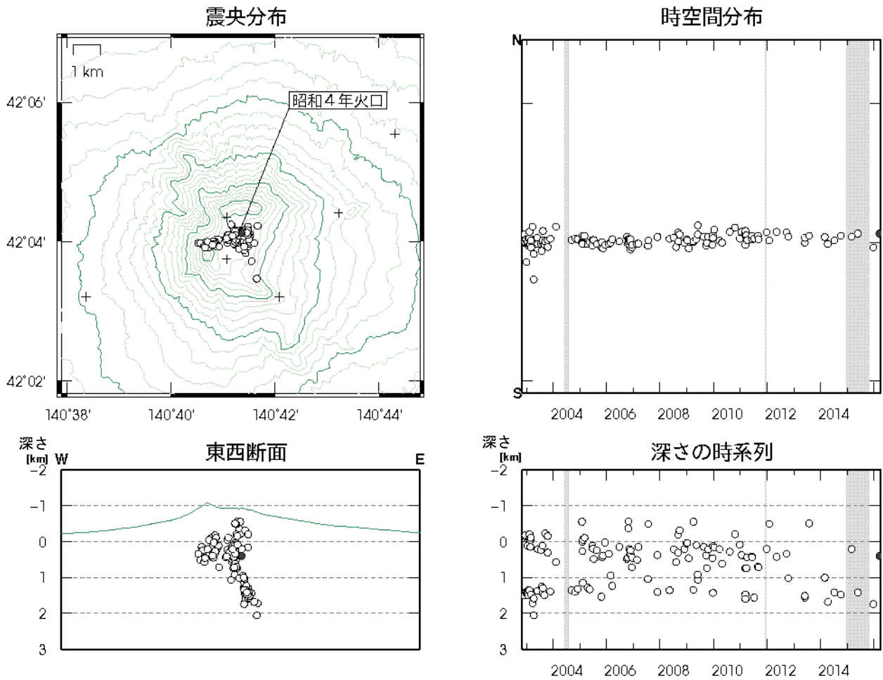
図4 北海道駒ヶ岳 火山性地震の震源分布（2002年12月～2016年3月） 灰色の期間は一部観測点欠測のため震源の決定数減少や精度低下が見られます ○印：2002年12月～2016年2月の震源 ●印：2016年3月の震源 +印：地震観測点
