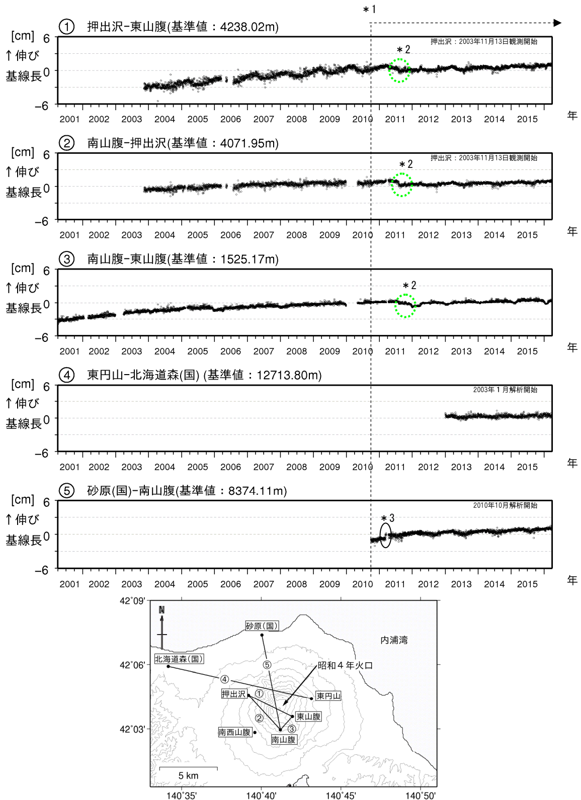
図5 北海道駒ヶ岳 GNSS連続観測による基線長変化（2001年4月～2016年3月）及び観測点配置図
