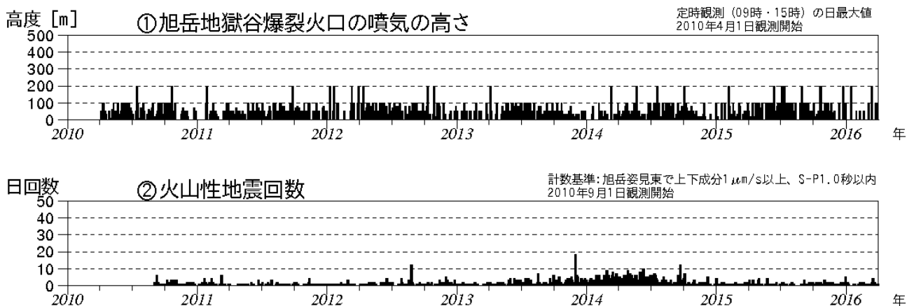
図 1 大雪山 火山活動経過図（2010年 4 月～2016年 3 月）
