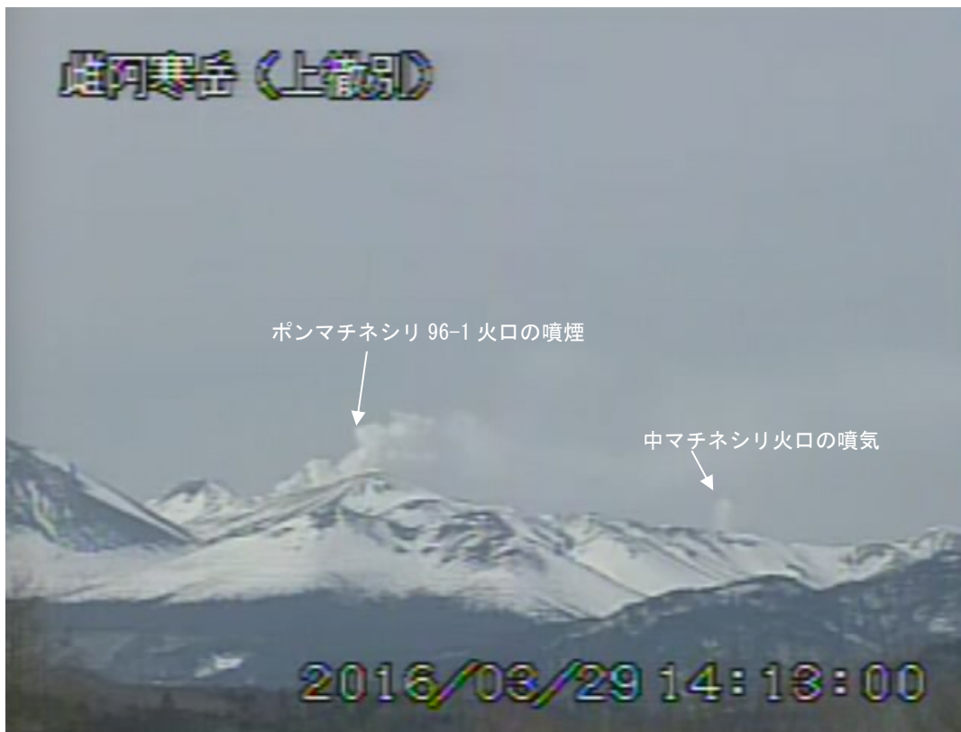
図3 雌阿寒岳 南東側から見た山体の状況 (3月29日、 かみてしべつ 上徹別遠望カメラによる)
