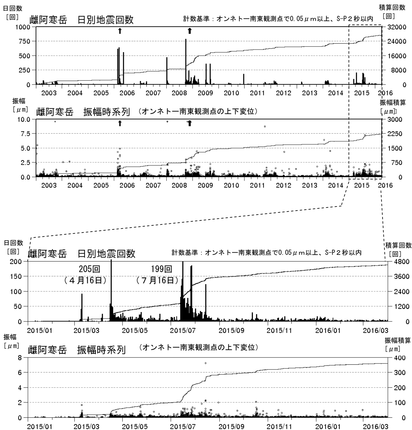
図5 雌阿寒岳 日別地震回数及び振幅時系列 上図：2003年1月1日～2016年3月31日 下図：2015年1月1日～2016年3月31日
