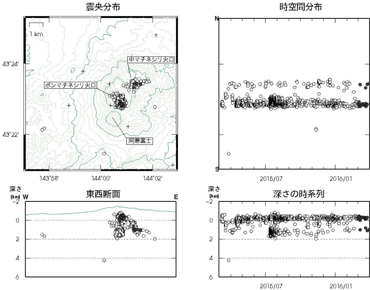
図 6 雌阿寒岳 火山性地震の震源分布 (2015年3月~2016年3月)
