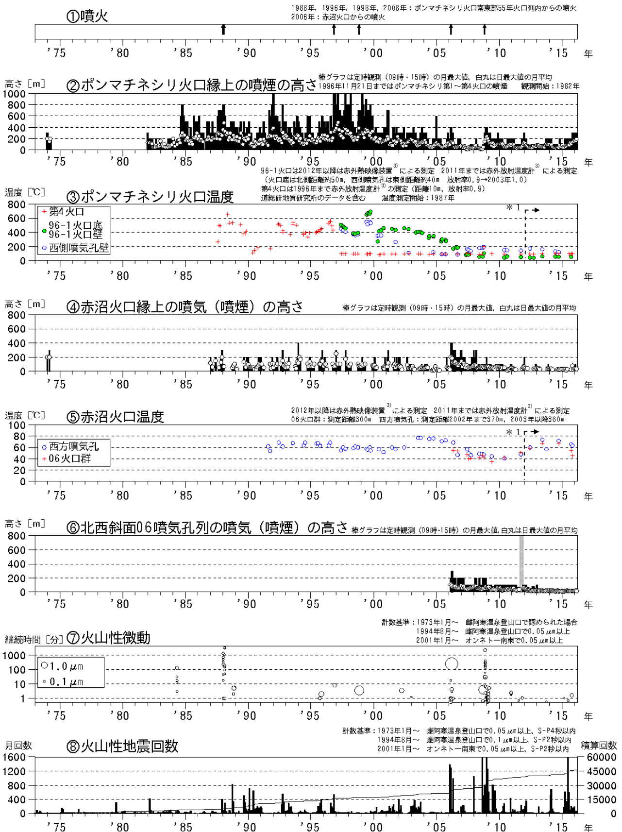
図1 雌阿寒岳 火山活動経過図（1973年1月～2016年3月）
