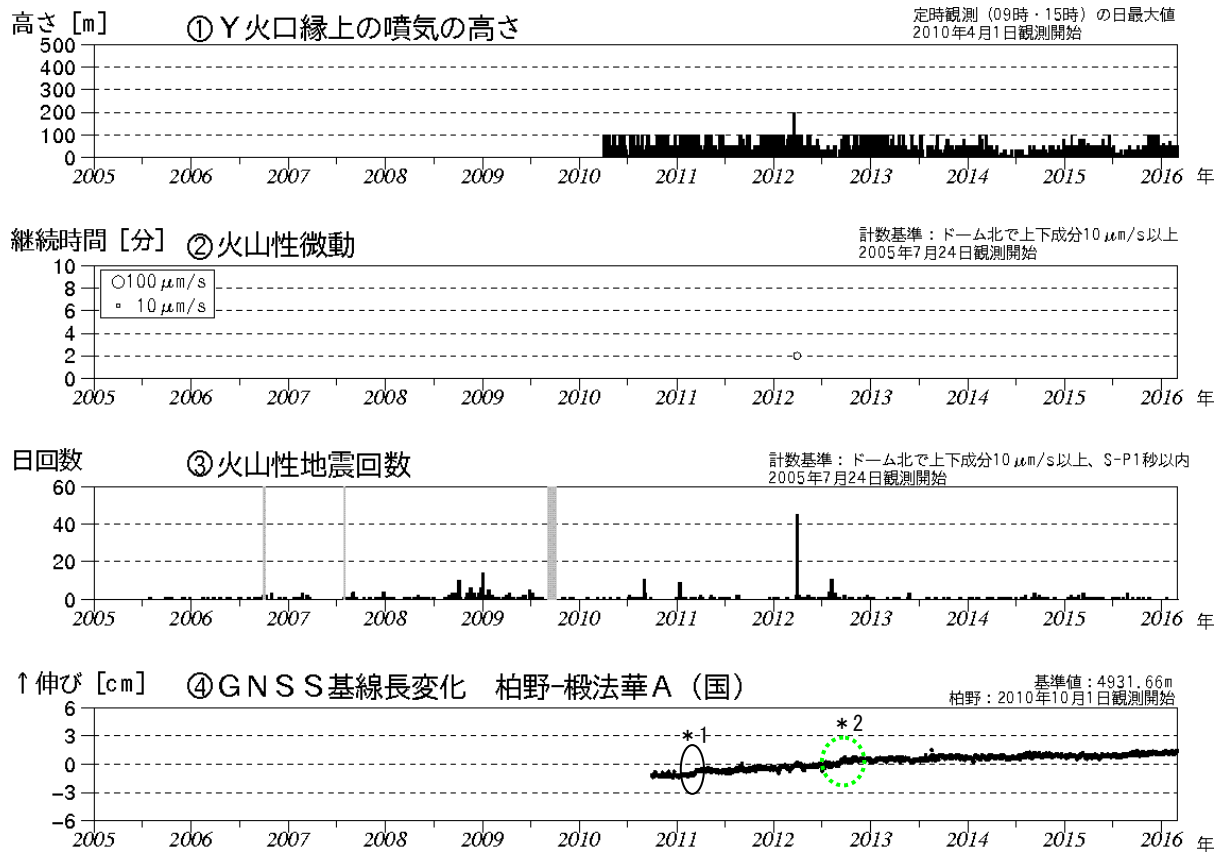
図2 恵山 火山活動経過図（2005年7月～2016年2月）
