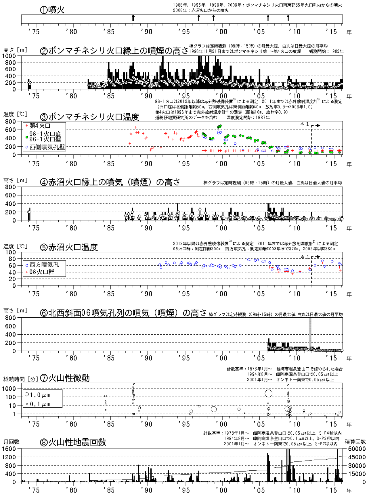
図1 雌阿寒岳 火山活動経過図（1973年1月～2016年2月）
