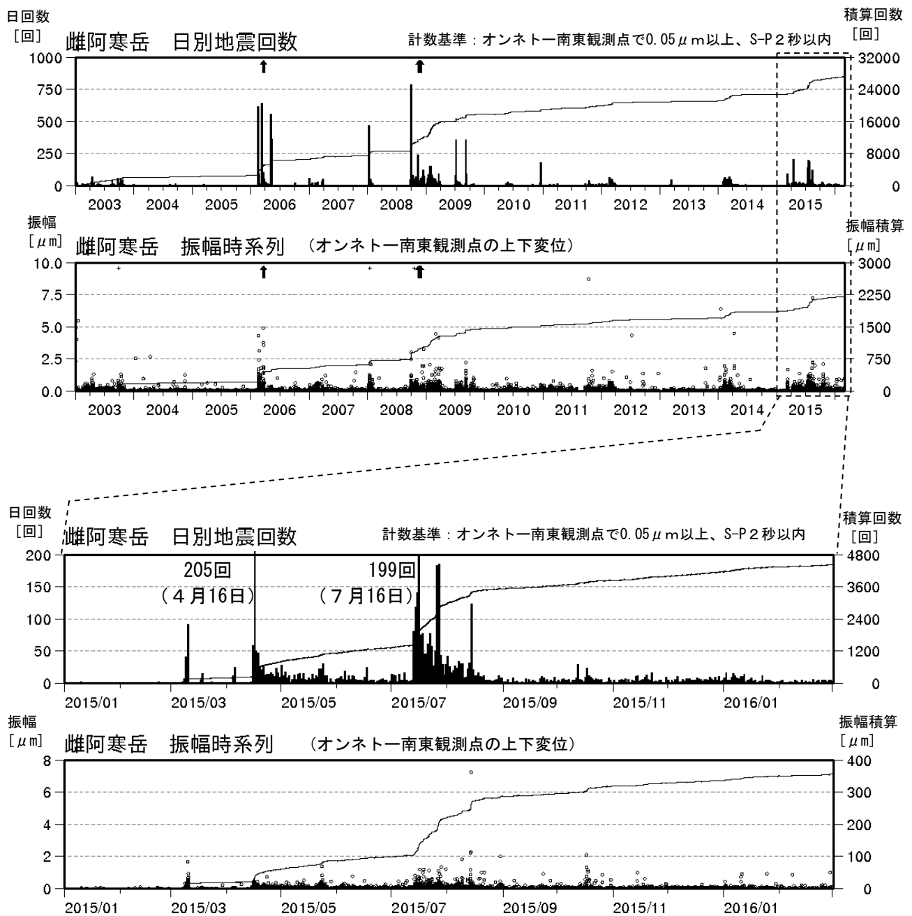
図5 雌阿寒岳 日別地震回数及び振幅時系列 上図：2003年1月1日～2016年2月29日 下図：2015年1月1日～2016年2月29日
