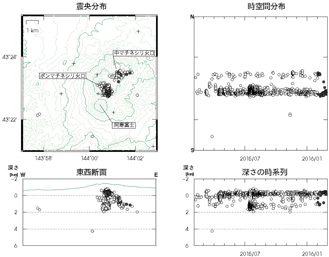
図 6 雌阿寒岳 火山性地震の震源分布（2015年2月～2016年2月）
