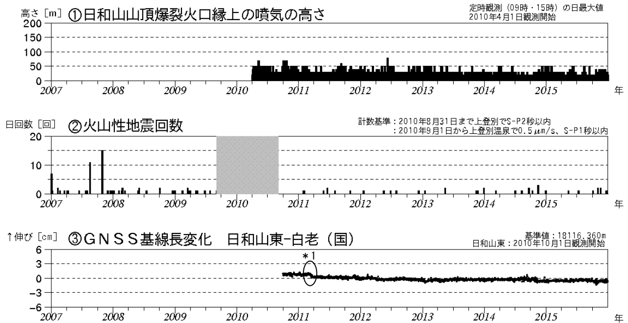
図2 倶多楽 火山活動経過図（2007年1月～2015年12月）
