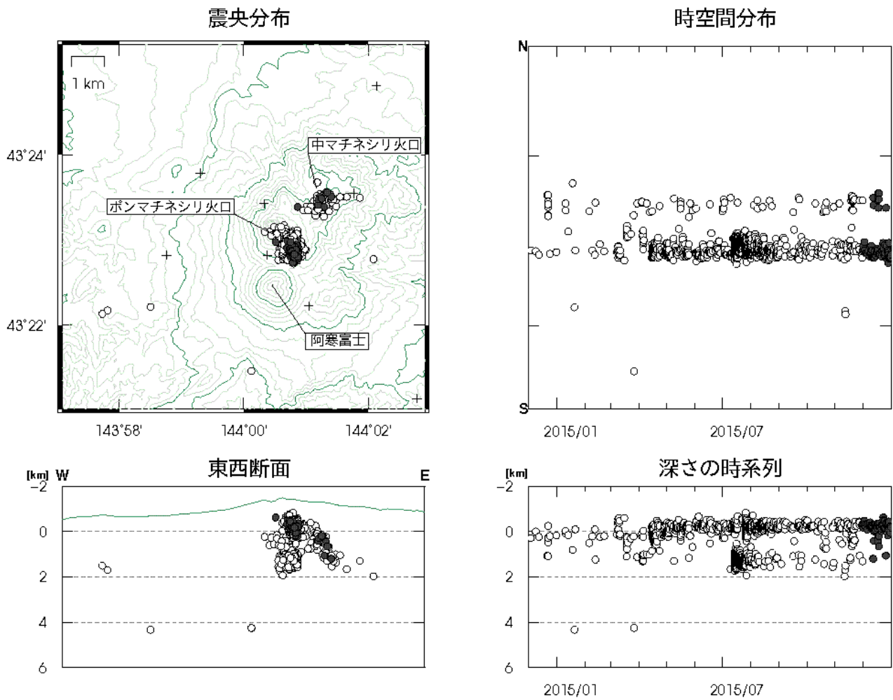
図 6 雌阿寒岳 火山性地震の震源分布（2014年12月～2015年12月）
